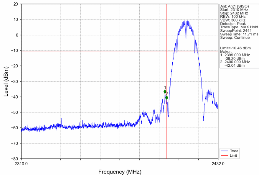
802.11b_LCH_2412MHz_Ant1 (SISO)_NTNV
