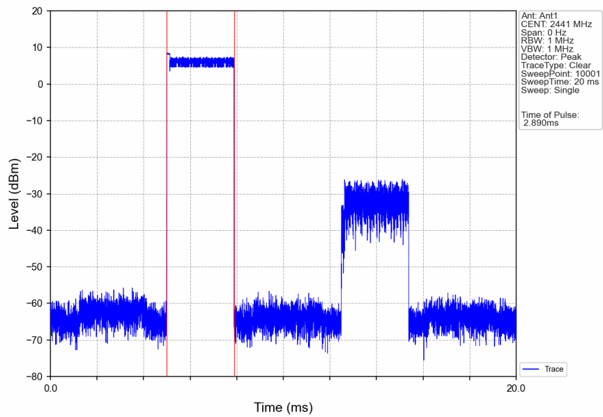
Pi/4DQPSK_2DH5_HOPP_Ant1_NTNV
