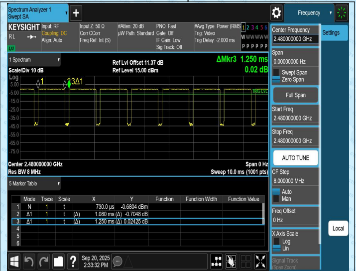
NTNV-BLE_2M-Ant1-2480
