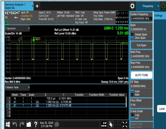
NTNV-BLE_2M-Ant1-2440
