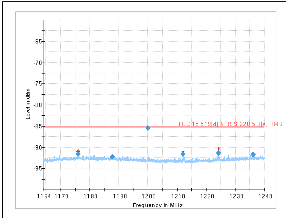
Plot 11: 1164 MHz to 1240 MHz §15.519 (d), UWB test mode
