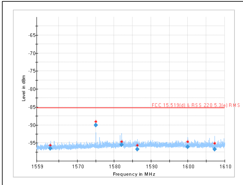
Plot 12: 1559 MHz to 1610 MHz §15.519 (d), UWB test mode
