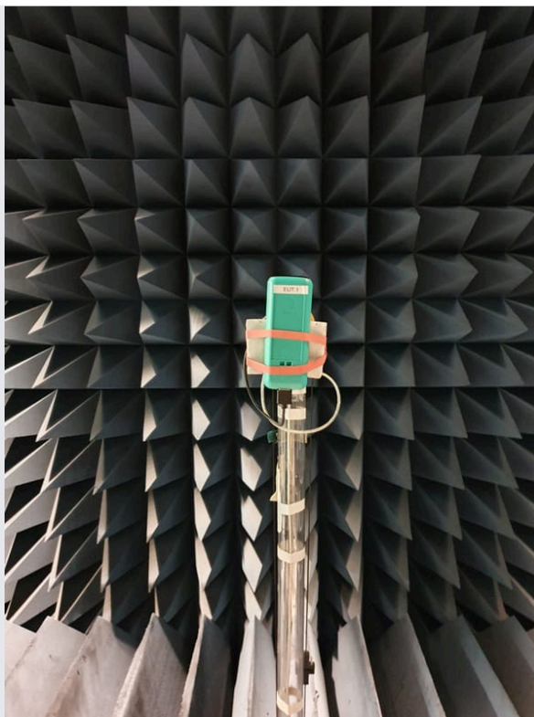
Photo 6 EUT 1
