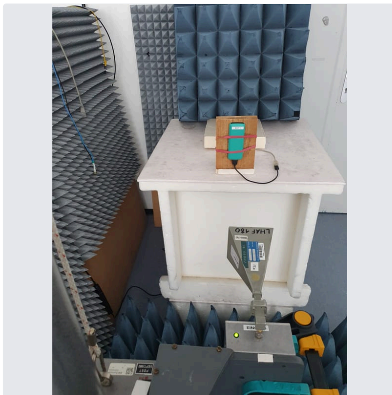
Photo 9 EUT 1
