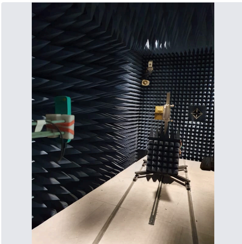
Photo 7 EUT 1
