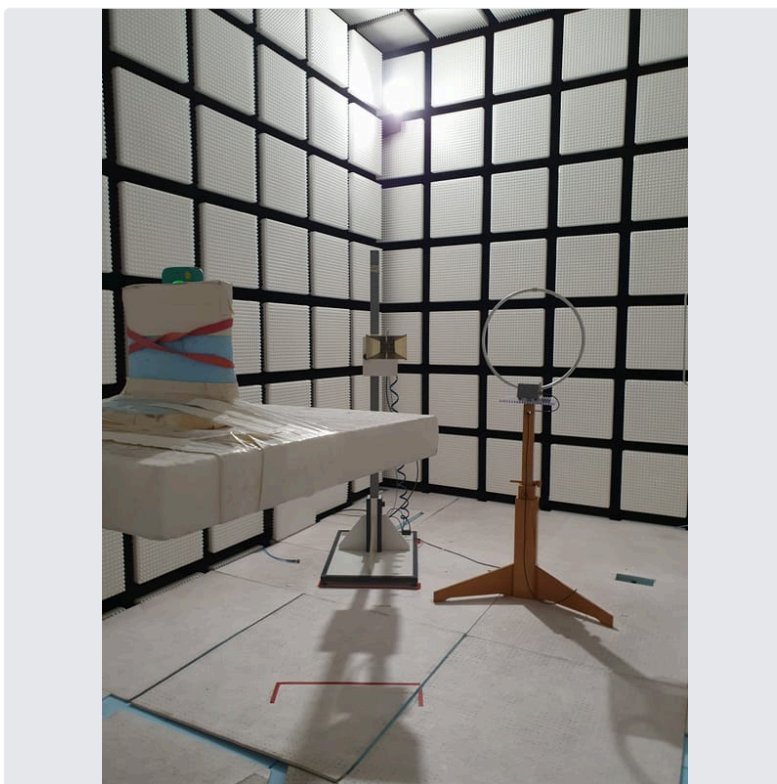
Photo 4 EUT 1
