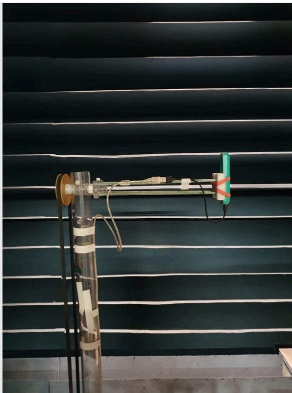
Photo 5 EUT 1
