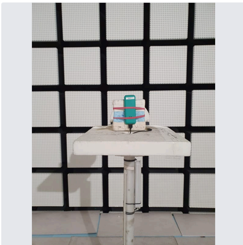
Photo 2 EUT 1
