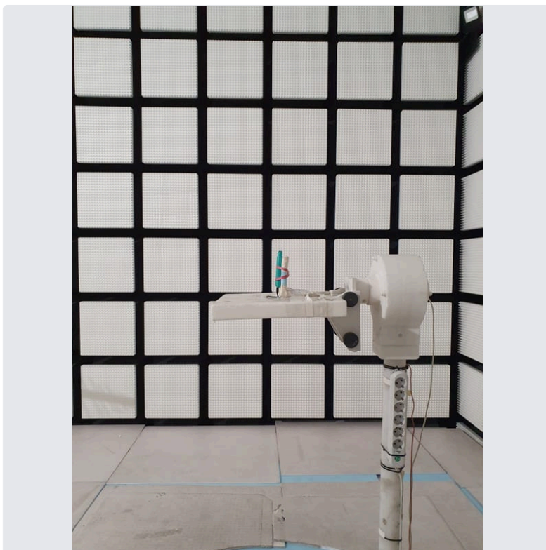
Photo 1 EUT 1
