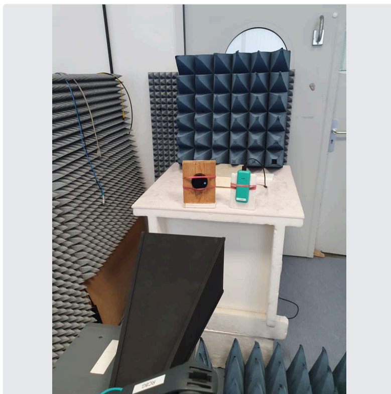
Photo 10 EUT 1+AE 1
