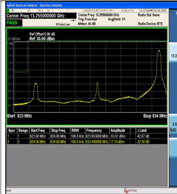
Band26(824-849)-10MHz-QPSK-26990-1RB#0-P ASS
