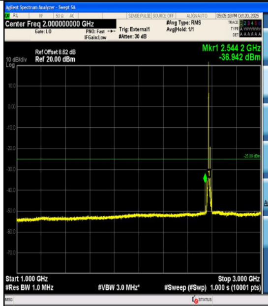
Band38-15MHz-QPSK-37825-1RB#0-18000~27 000-PASS
