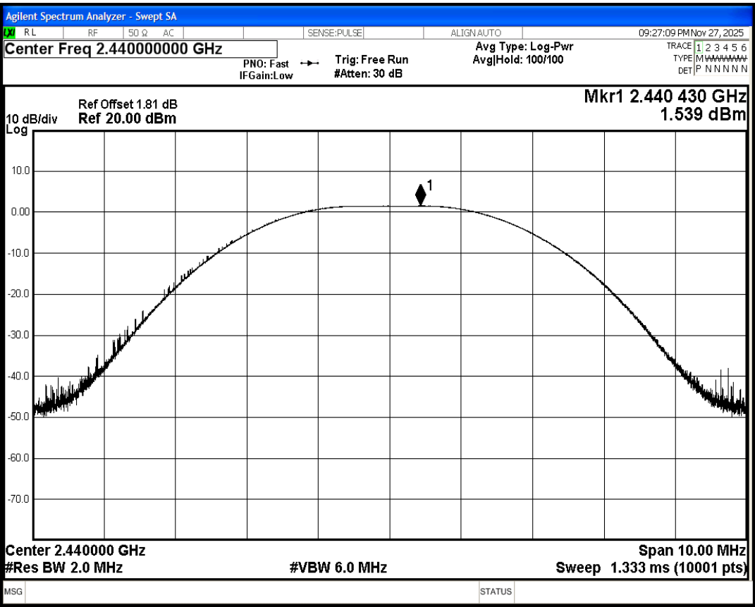
Power NVNT BLE 2M 2440MHz Ant1
