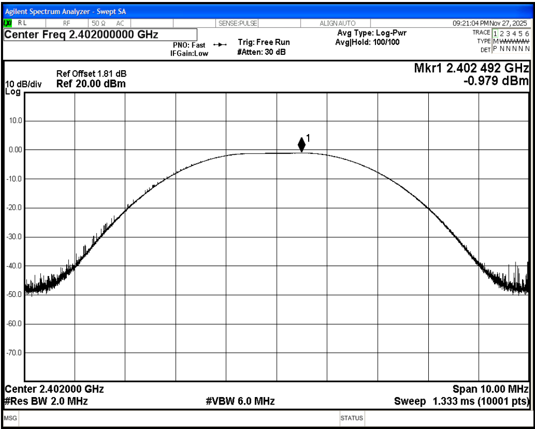
Power NVNT BLE 2M 2402MHz Ant1
