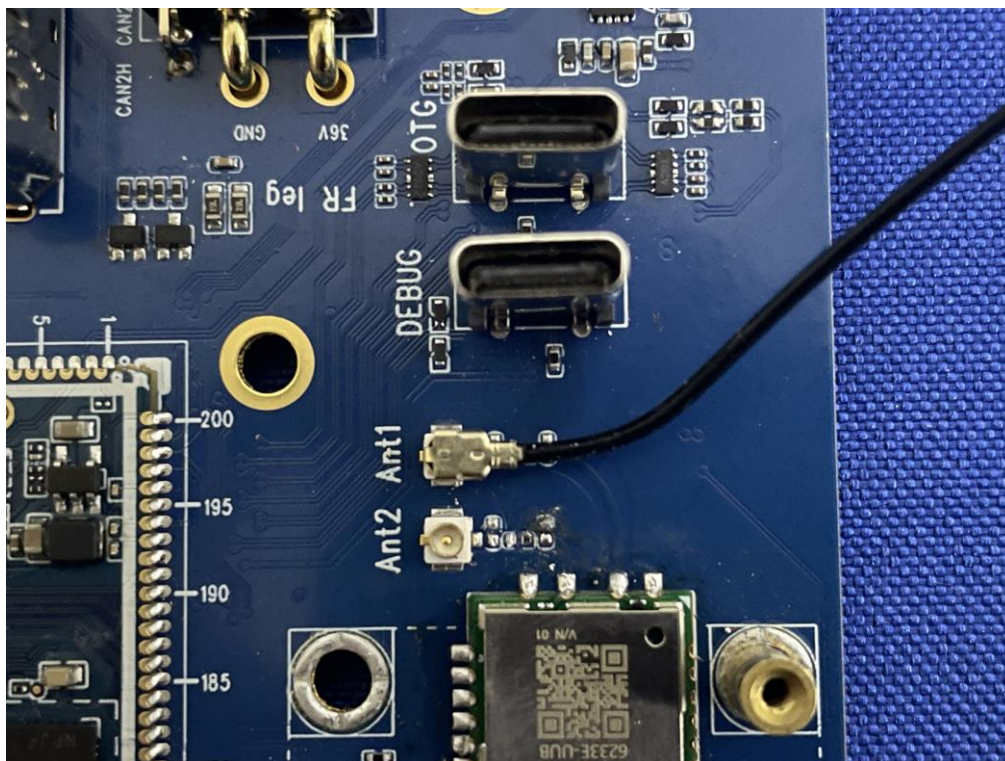
BR&EDR/BLE/WIFI Antenna Jack
