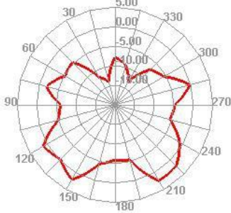
2500.000MHz E2
