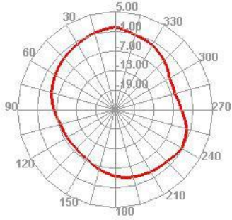
2500.000MHz H
