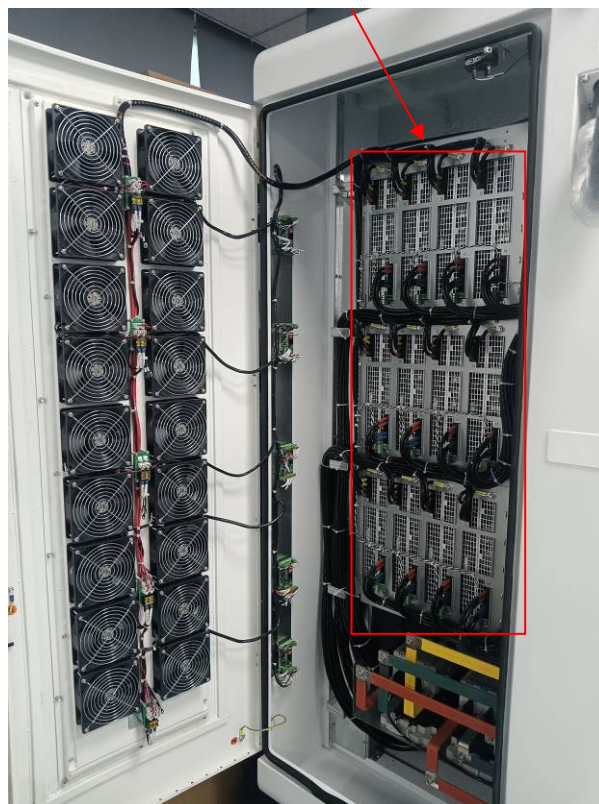
Power Module
