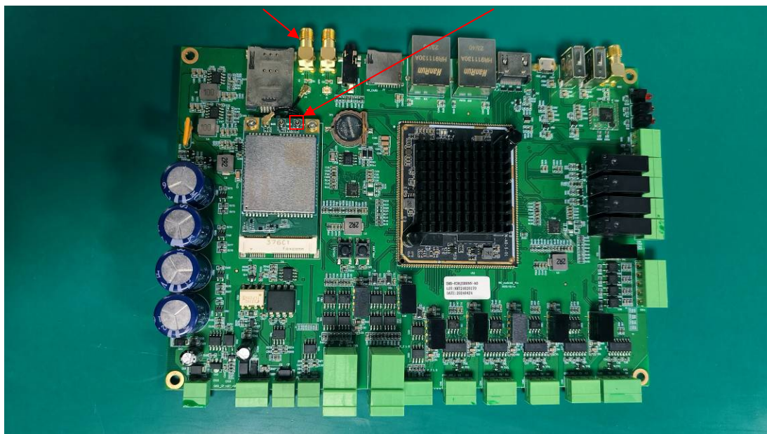
WWAN DIV antenna
