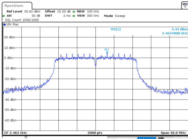
802.11n20_2462MHz
