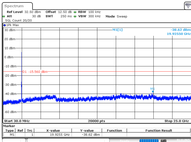
802.11n20_2462MHz
