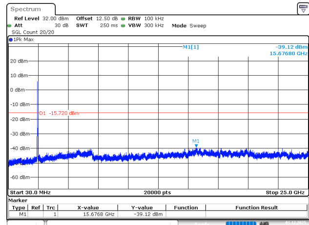
802.11n20_2437MHz
