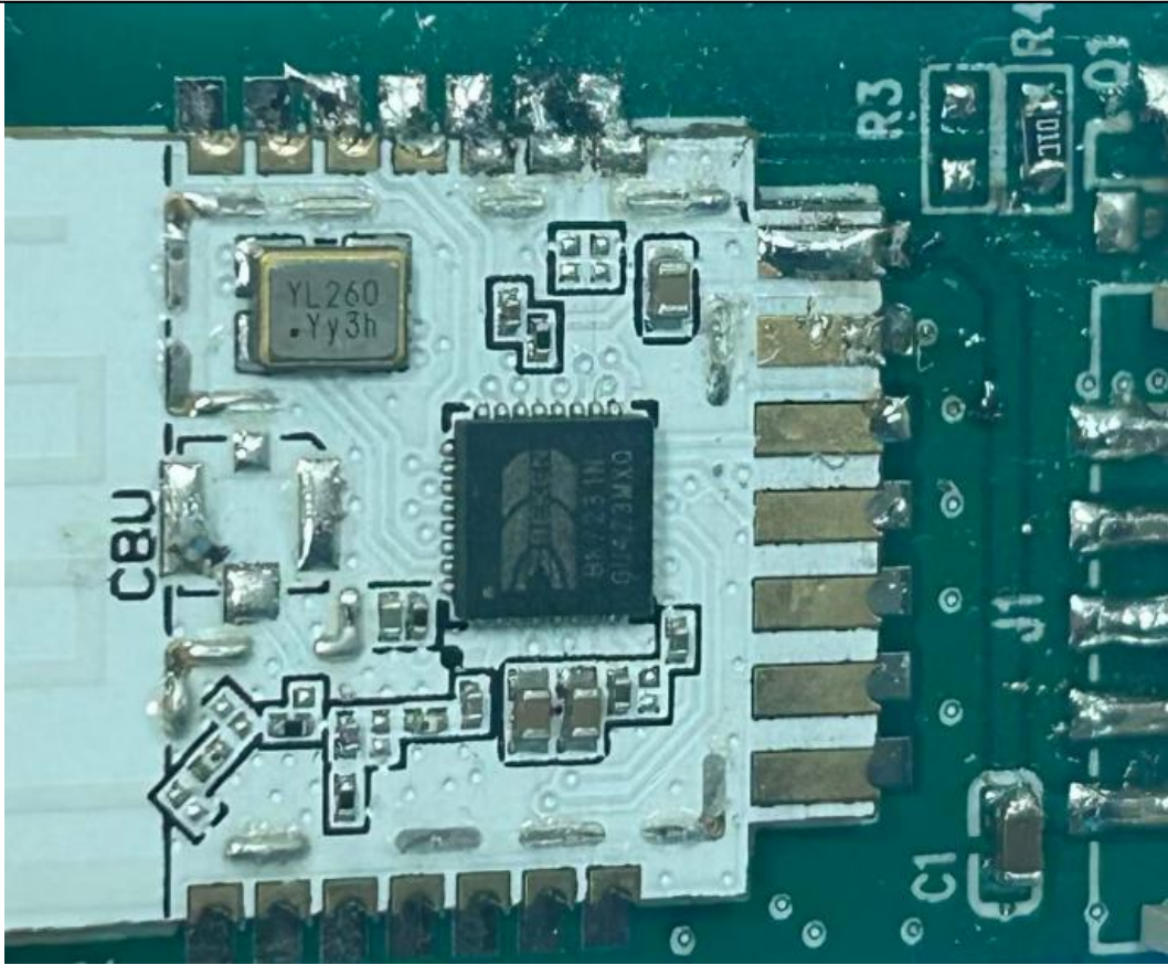
EUT Photo
