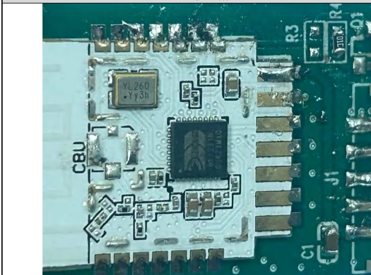
EUT Photo
