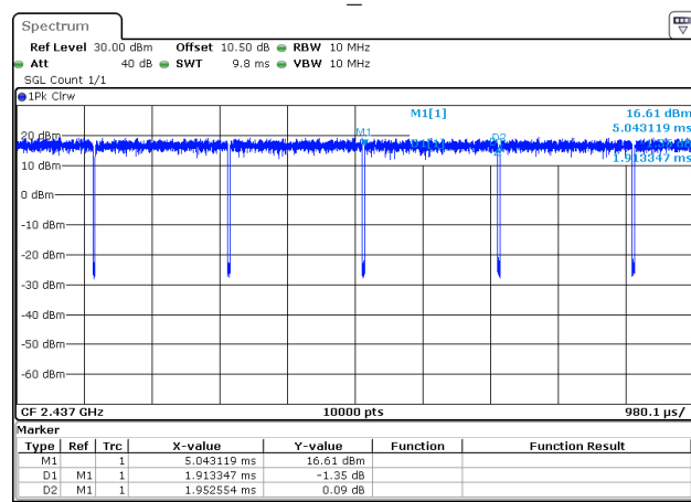
802.11n20_2437MHz
