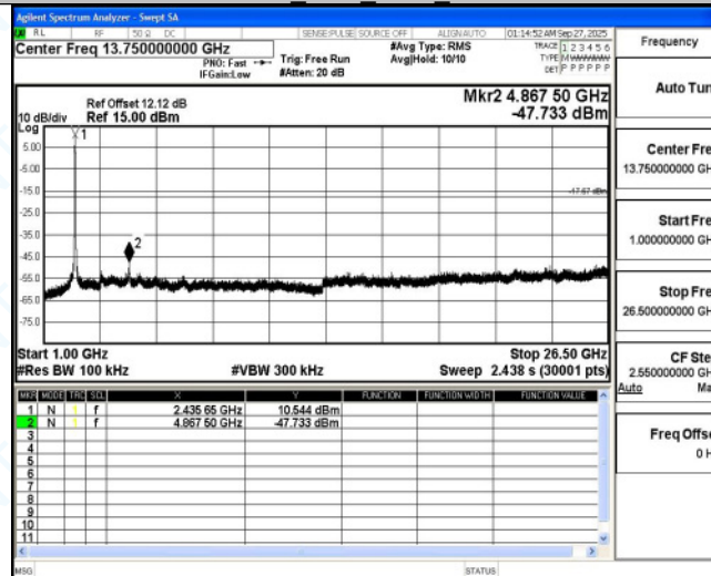
11N40MIMO_Ant1_2452_0~Reference
