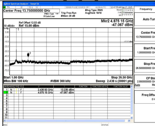
11N20MIMO_Ant2_2437_0~Reference
