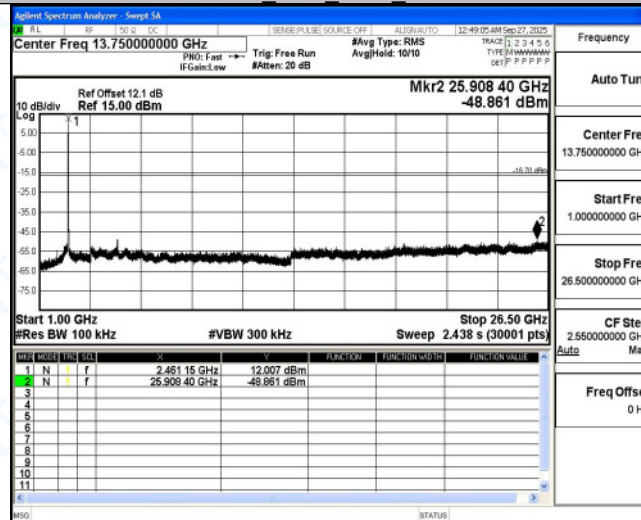
11N20MIMO_Ant2_2462_0~Reference
