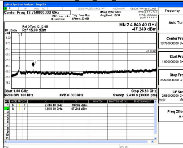
11N40MIMO_Ant1_2437_0~Reference
