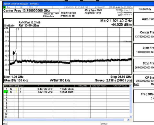
11AX20MIMO Ant2 2437 0~Reference
