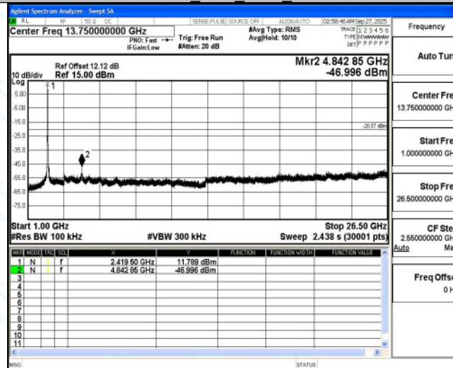
11AX40MIMO Ant1 2437 0~Reference
