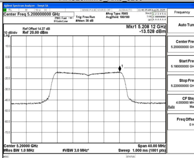
11AC20MIMO_Ant4_5200
