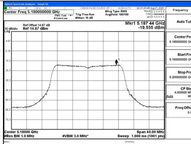
11N20MIMO Ant4 5180
