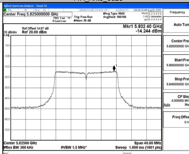
11A Ant6 5825
