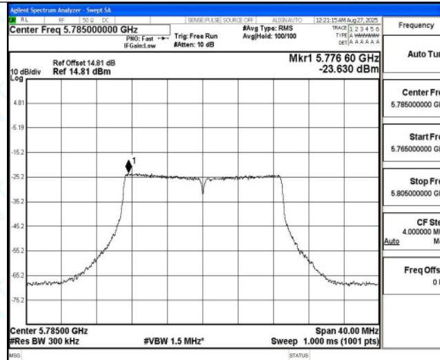
11AC20MIMO_Ant5_5785
