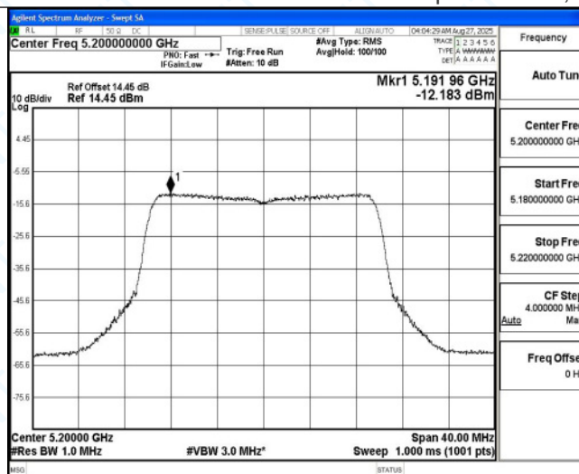
11AX20MIMO_Ant5_5200
