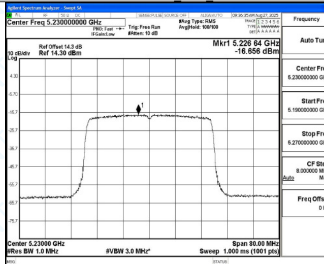
11AX40MIMO_Ant4_5230
