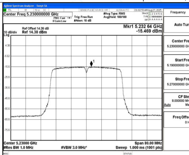
11AC40MIMO_Ant5_5230
