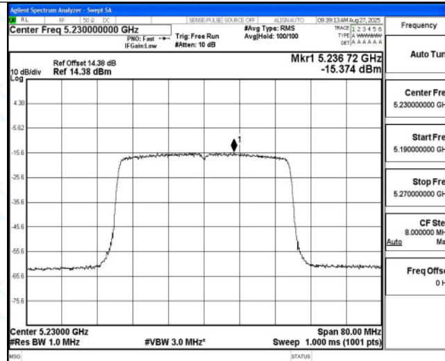
11AX40MIMO_Ant5_5230
