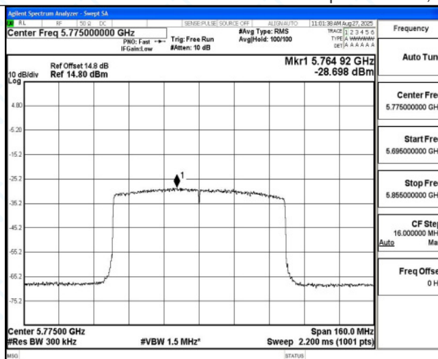
11AX80MIMO_Ant4 5775
