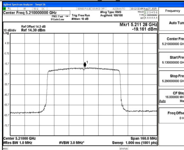
11AX80MIMO_Ant3_5210
