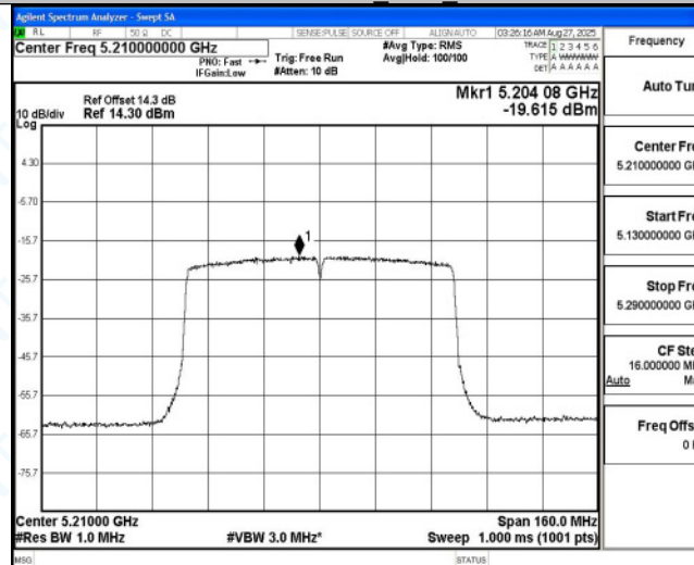
11AC80MIMO_Ant4_5210
