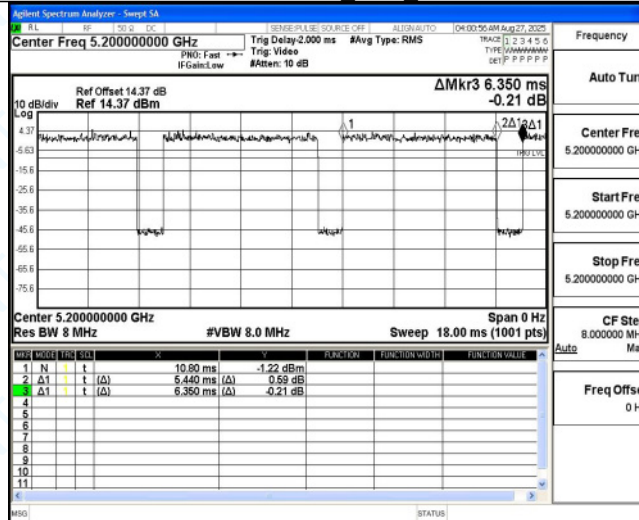
11AX20MIMO_Ant4_5200
