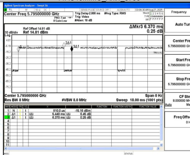
11AC40MIMO_Ant5_5795
