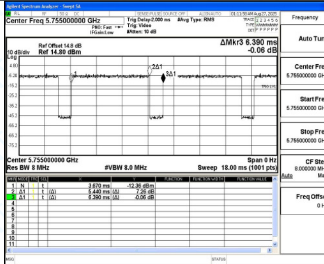
11AC40MIMO_Ant4 5755
