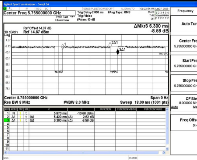
11AC40MIMO_Ant6 5755
