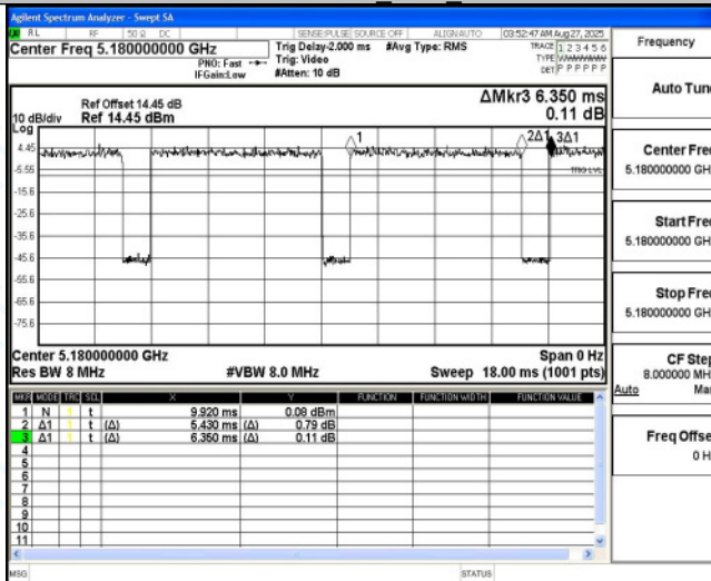
11AX20MIMO_Ant5_5180
