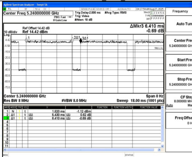
11AX20MIMO_Ant6 5240
