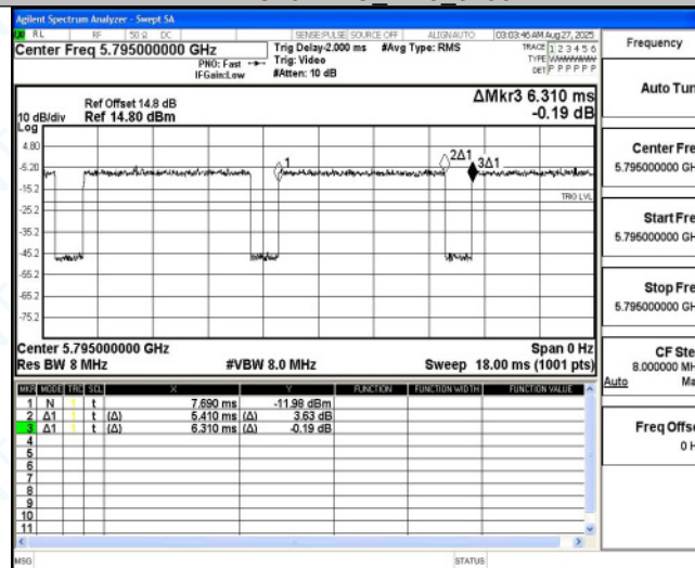
11AC40MIMO_Ant4_5795
