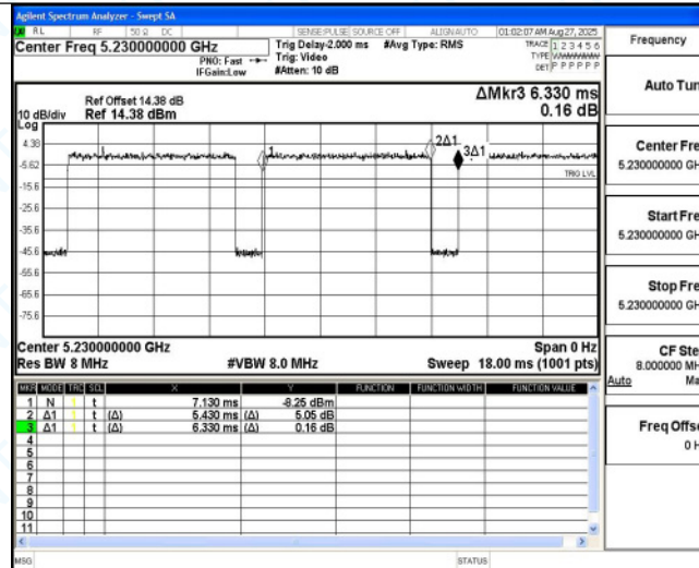
11AC40MIMO_Ant5_5230
