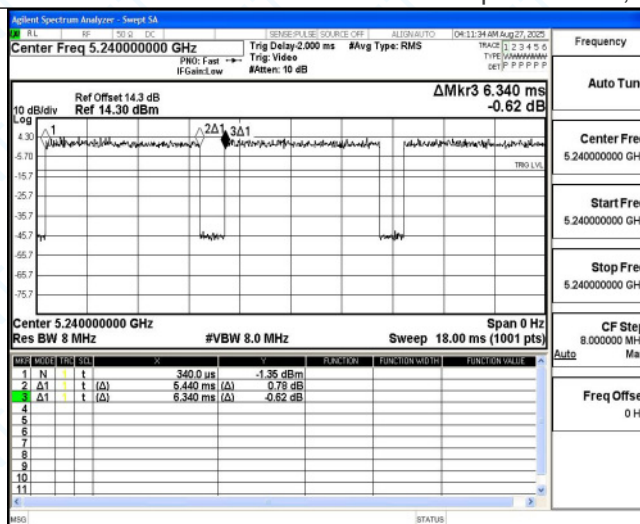
11AX20MIMO_Ant4 5240
