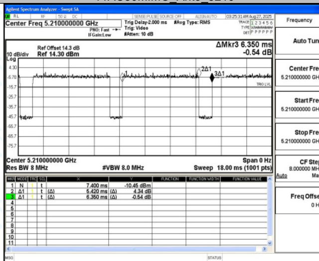
11AC80MIMO_Ant4_5210
