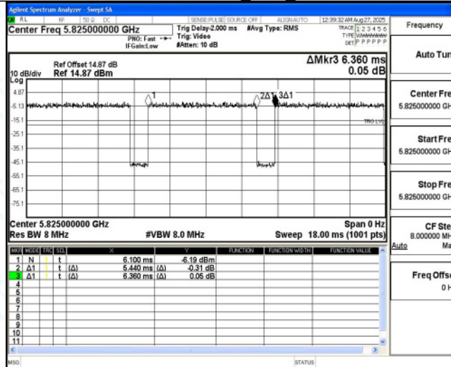
11AC20MIMO_Ant6 5825
