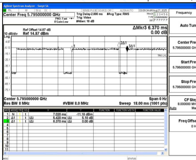
11AC40MIMO_Ant6_5795
