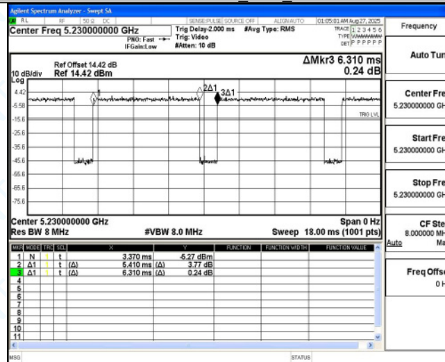
11AC40MIMO_Ant6_5230
