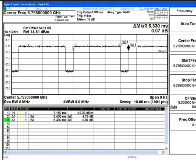
11AC40MIMO_Ant5 5755
