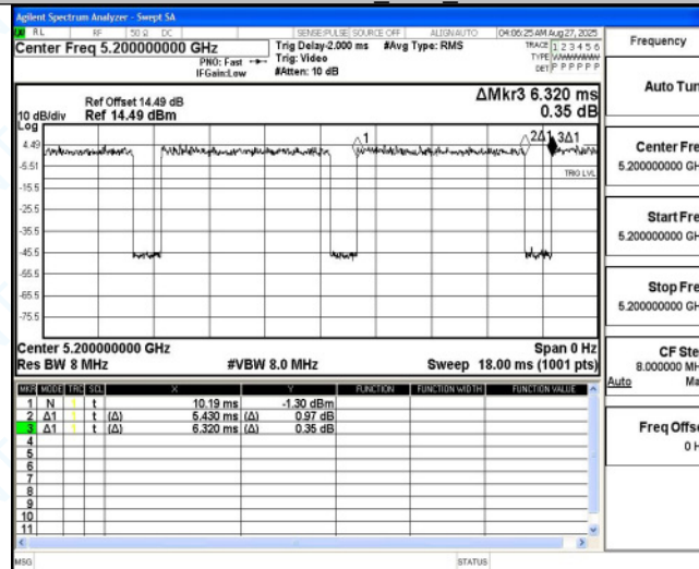
11AX20MIMO_Ant6_5200
