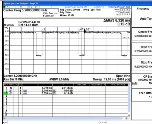
11AX20MIMO_Ant5_5200
