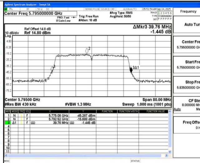
11N40MIMO Ant4 5795
