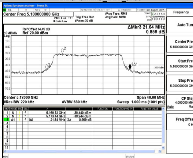
11AC20MIMO_Ant5_5180
