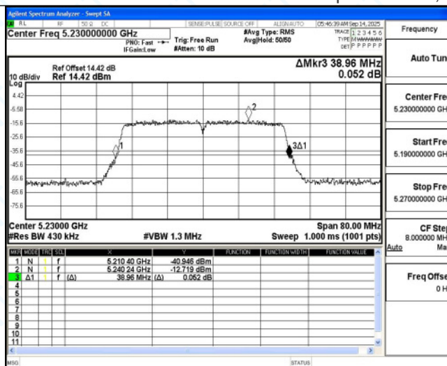
11N40MIMO Ant6 5230
