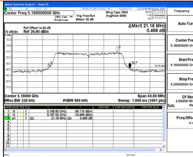
11AC20MIMO_Ant6_5180
