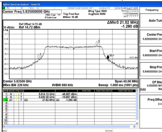
11AC20MIMO_Ant4 5825
