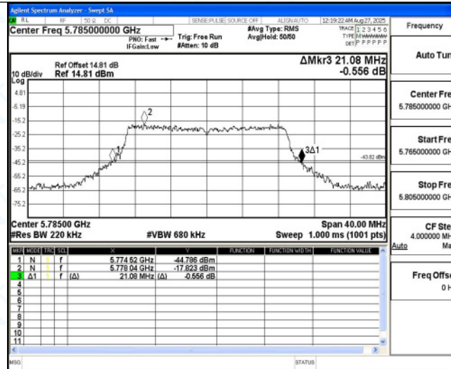
11AC20MIMO_Ant5_5785
