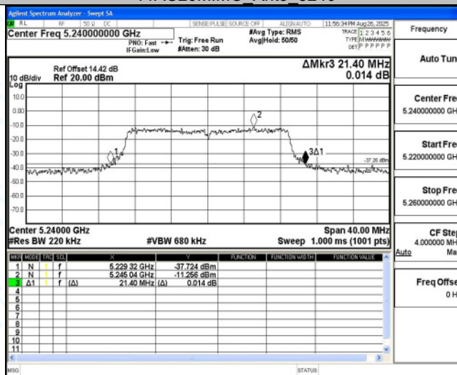
11AC20MIMO_Ant6 5240
