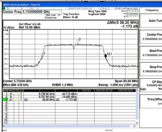
11N40MIMO Ant4 5755
