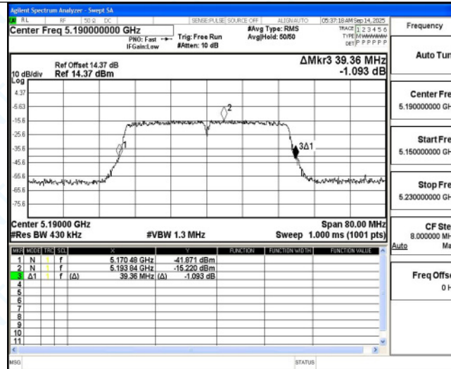
11N40MIMO Ant4 5190
