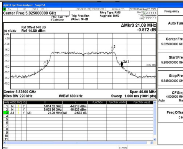
11AC20MIMO_Ant5 5825
