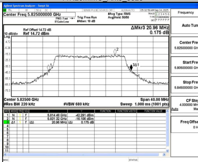
11N20MIMO Ant4 5825
