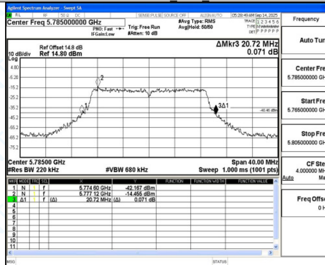
11N20MIMO Ant4 5785
