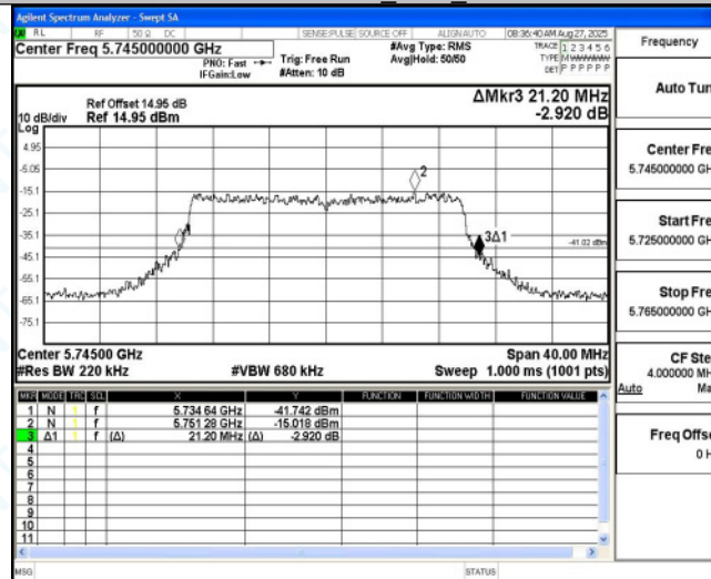
11AC20MIMO_Ant4_5745
