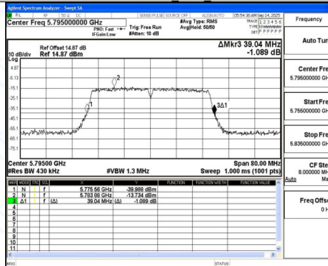
11N40MIMO Ant6 5795
