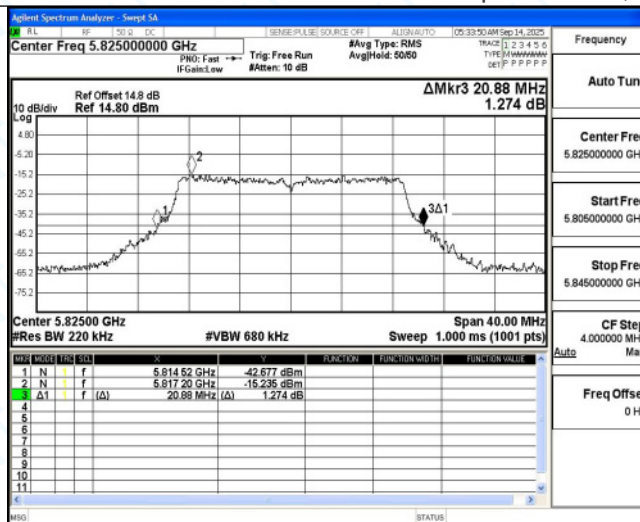
11N20MIMO Ant5 5825
