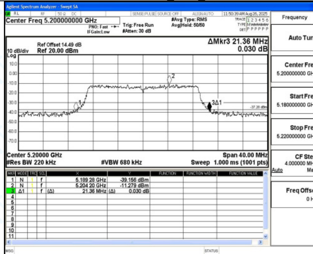
11AC20MIMO_Ant6_5200
