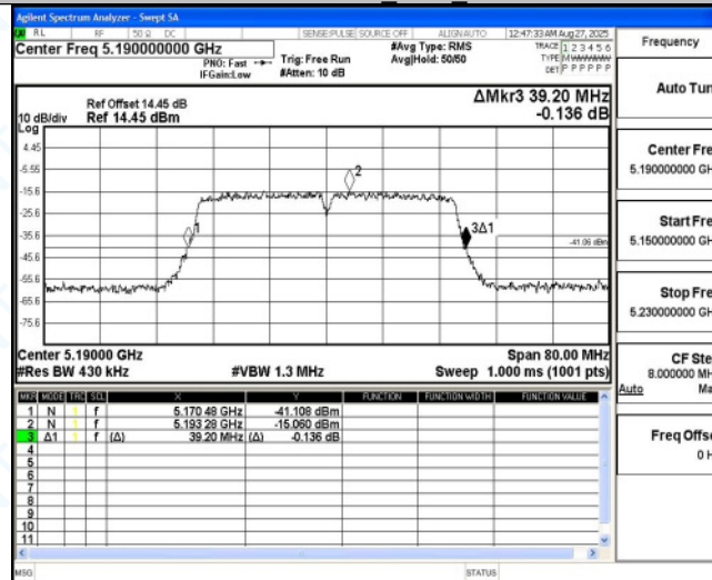
11AC40MIMO_Ant5_5190
