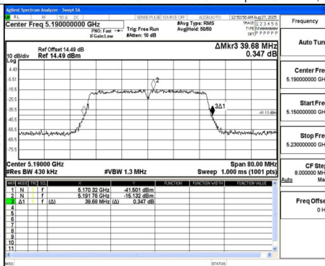
11AC40MIMO_Ant6_5190
