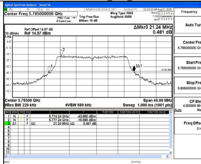
11AC20MIMO_Ant6_5785
