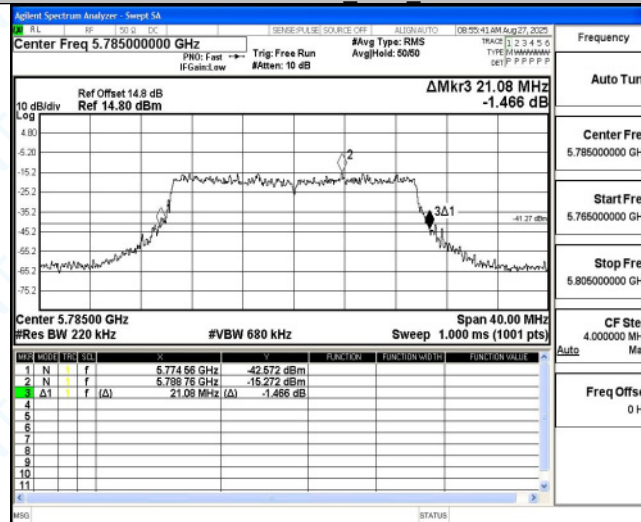
11AC20MIMO_Ant4_5785
