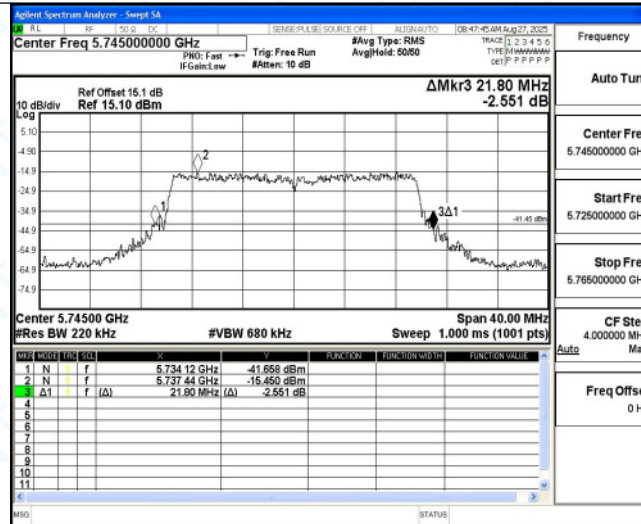
11AC20MIMO_Ant6_5745
