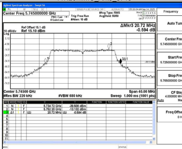
11N20MIMO Ant6 5745
