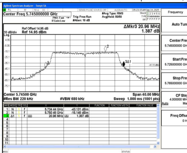
11N20MIMO Ant4 5745
