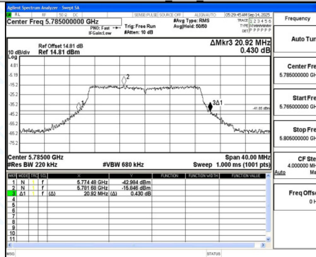
11N20MIMO Ant5 5785
