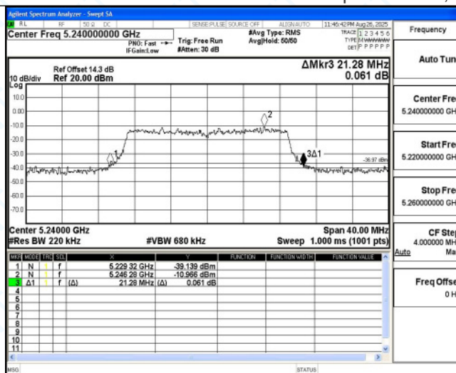
11AC20MIMO_Ant4 5240
