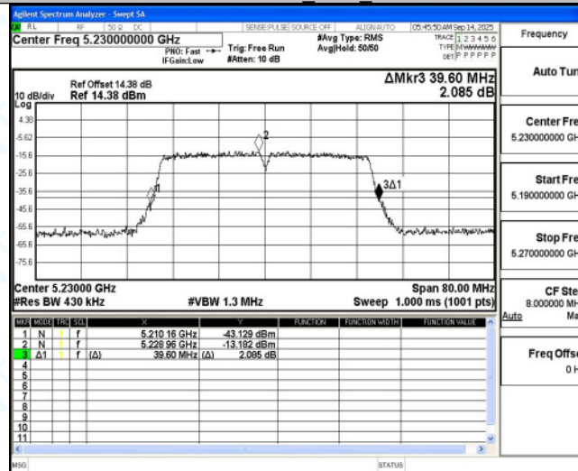
11N40MIMO Ant5 5230
