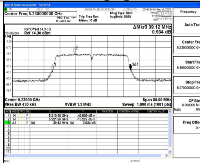
11N40MIMO Ant4 5230
