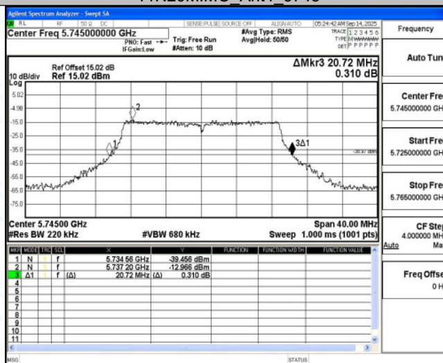
11N20MIMO Ant5 5745
