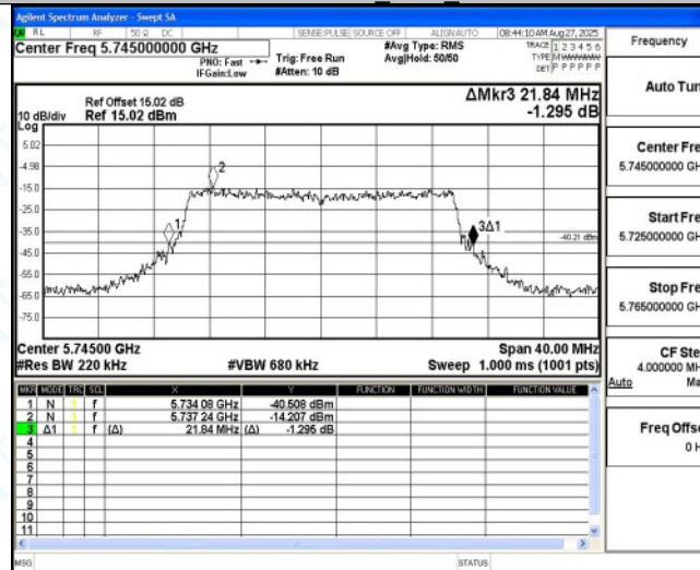
11AC20MIMO_Ant5_5745
