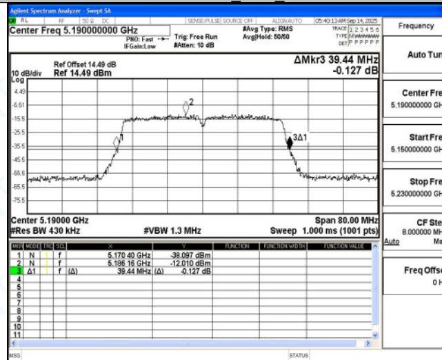
11N40MIMO Ant6 5190
