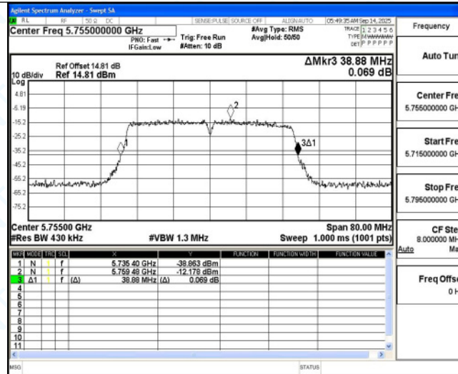
11N40MIMO Ant5 5755
