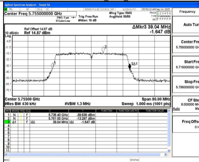
11N40MIMO Ant6 5755
