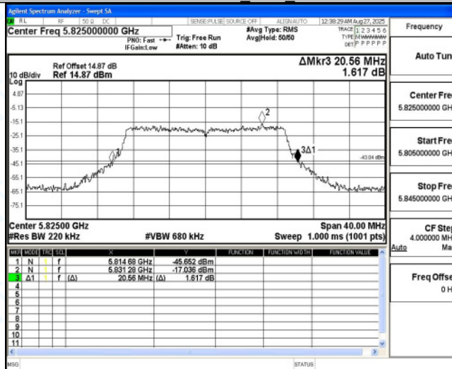
11AC20MIMO_Ant6 5825
