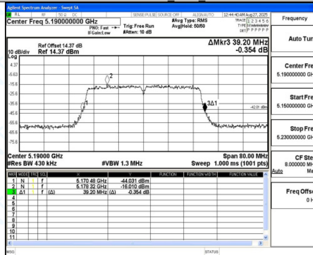
11AC40MIMO_Ant4_5190
