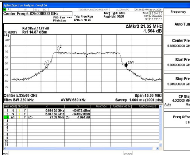
11N20MIMO Ant6 5825
