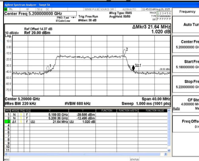
11AC20MIMO_Ant4_5200
