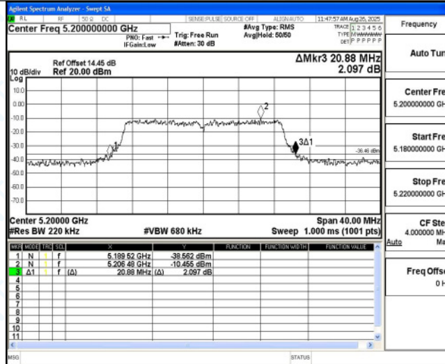
11AC20MIMO_Ant5_5200
