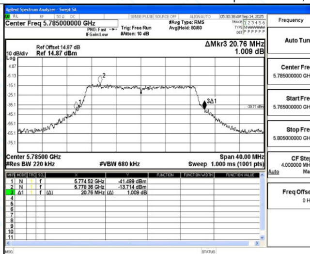
11N20MIMO Ant6 5785
