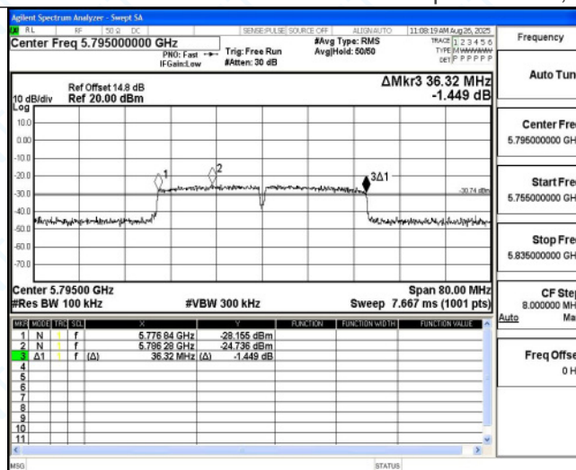
11N40MIMO Ant4 5795
