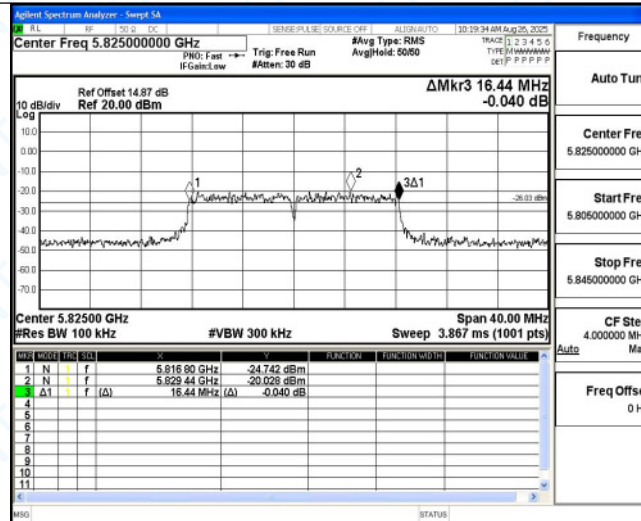
11N20MIMO Ant6 5825
