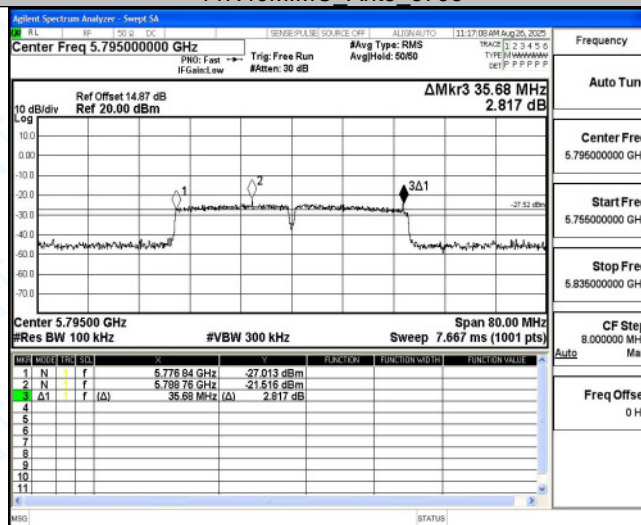
11N40MIMO Ant6 5795
