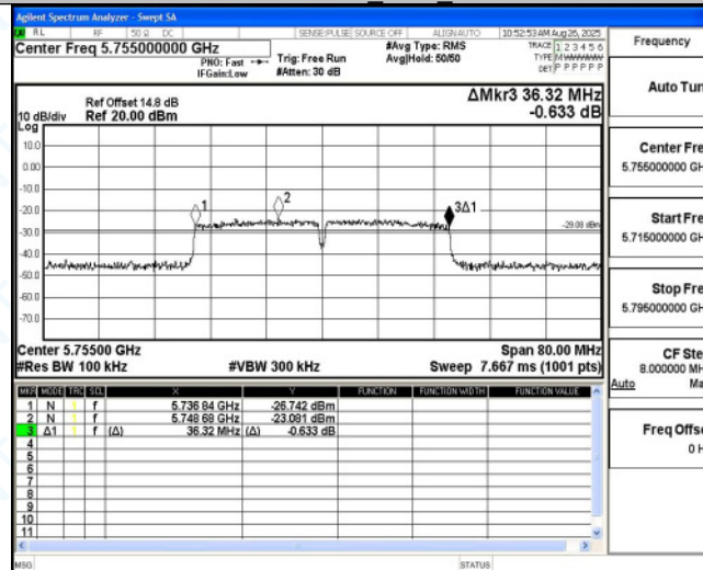
11N40MIMO Ant4 5755
