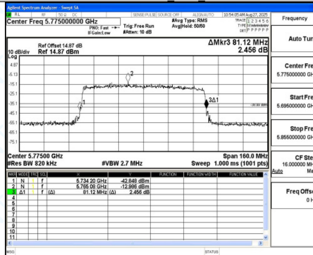
11AX80MIMO_Ant6 5775
