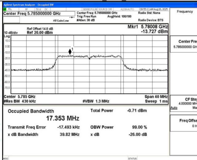
11N20MIMO Ant4 5785
