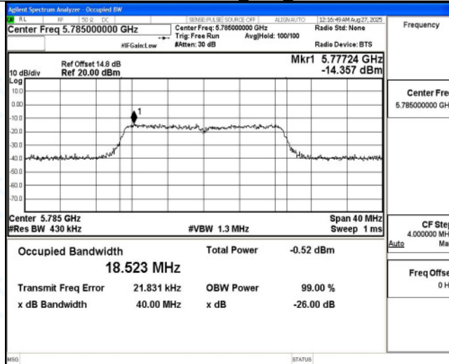
11AC20MIMO_Ant4_5785
