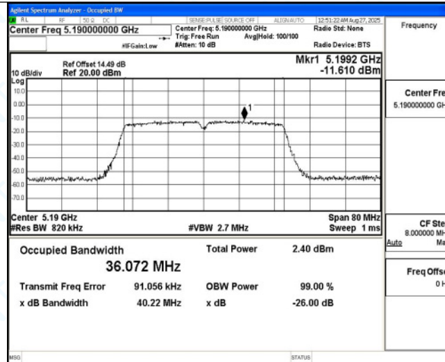
11AC40MIMO_Ant6_5190
