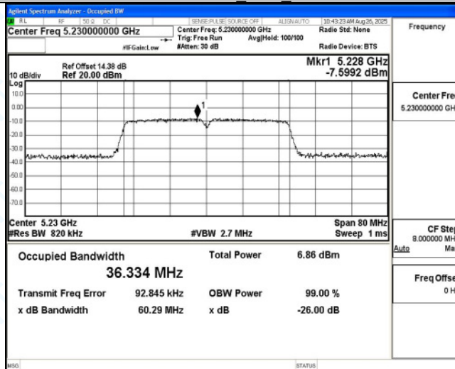
11N40MIMO Ant5 5230
