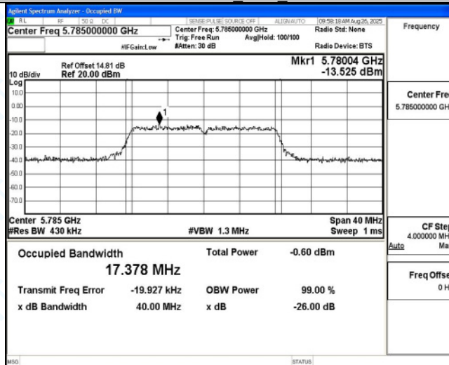
11N20MIMO Ant5 5785
