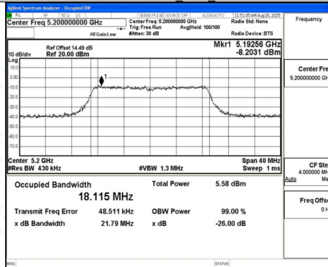
11AC20MIMO_Ant6_5200
