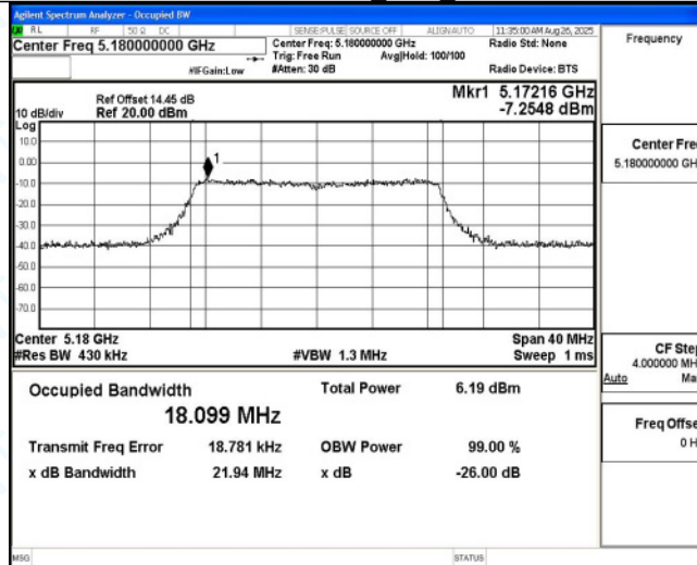
11AC20MIMO_Ant5_5180
