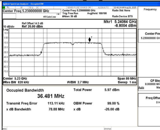
11N40MIMO Ant4 5230
