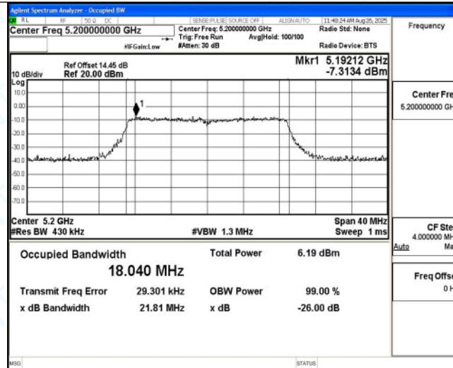
11AC20MIMO_Ant5_5200
