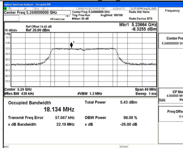
11AC20MIMO_Ant6 5240
