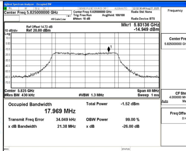
11AC20MIMO_Ant4 5825
