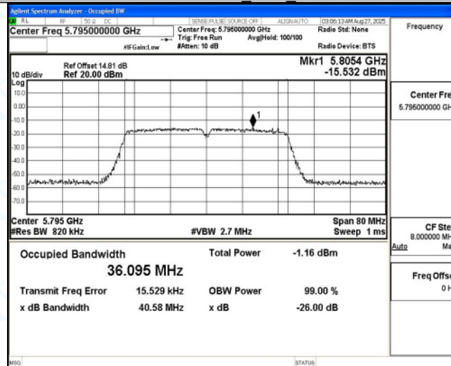
11AC40MIMO_Ant5_5795
