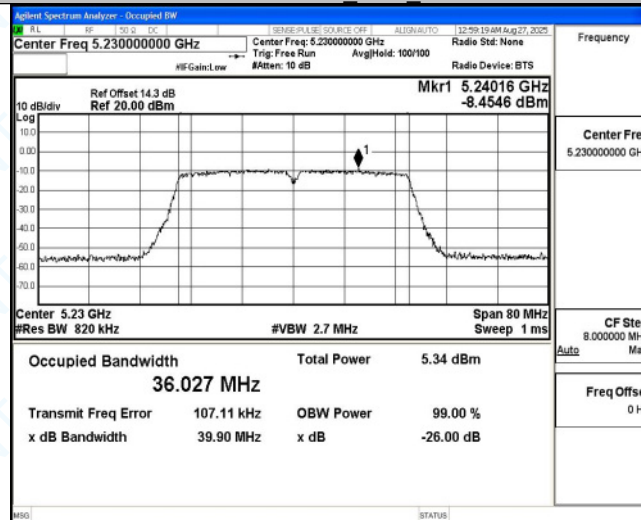
11AC40MIMO_Ant4_5230
