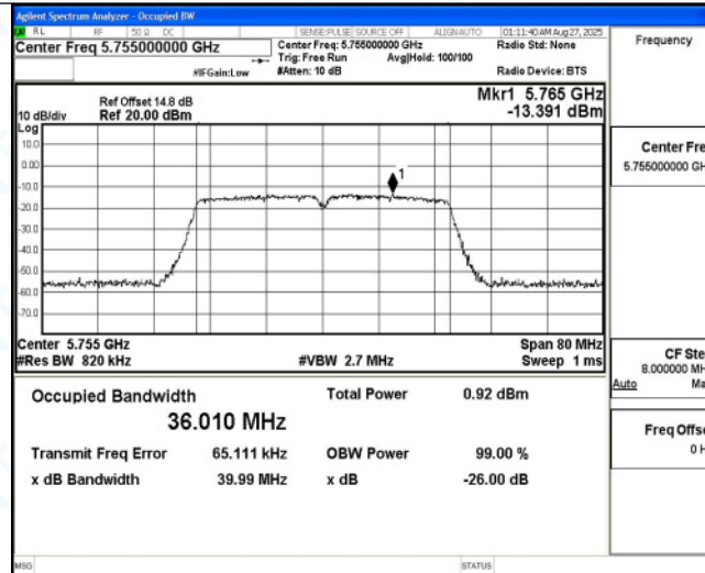
11AC40MIMO_Ant4 5755
