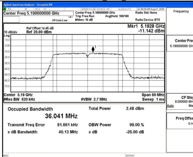
11AC40MIMO_Ant5_5190
