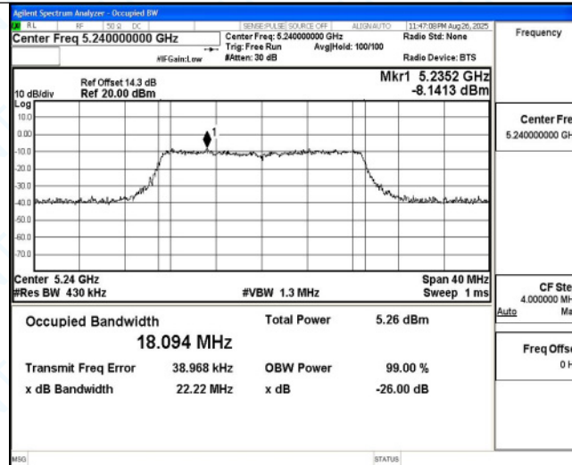
11AC20MIMO_Ant4 5240
