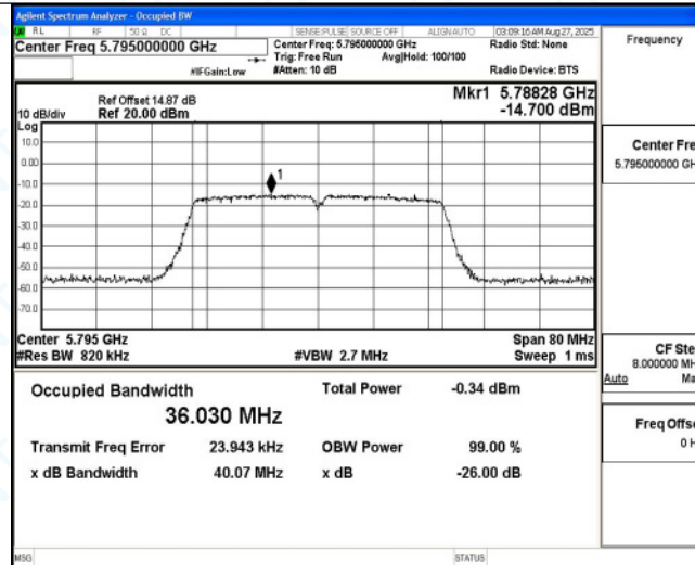
11AC40MIMO_Ant6_5795
