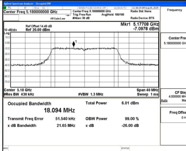
11AC20MIMO_Ant6_5180
