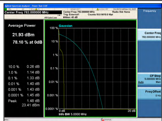
Band13-0.18-BPSK-23230-PASS
