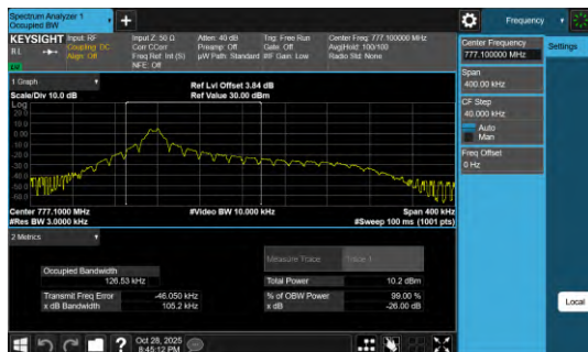
Band13-0.18-BPSK-23181-PASS
