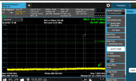
Band13-0.18-BPSK-23279-30-1000-PASS
