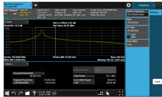
Band13-0.18-BPSK-23230-PASS
