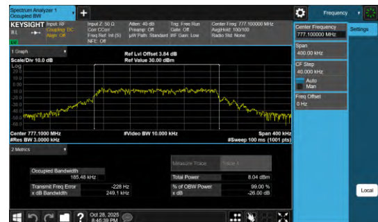
Band13-0.18-BPSK-23181-PASS
