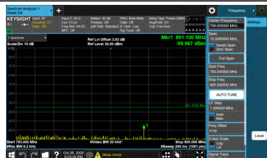
Band13-0.18-QPSK-23230-793-805-PASS
