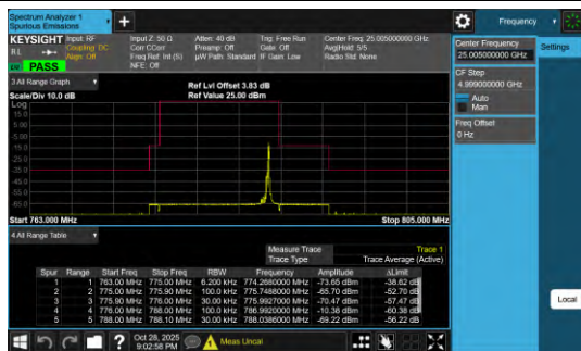
Band13-0.18-BPSK-23279-PASS
