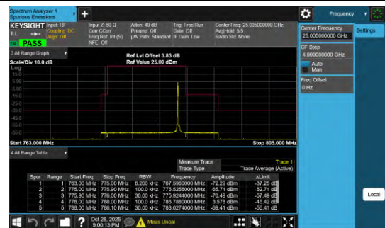
Band13-0.18-BPSK-23279-PASS
