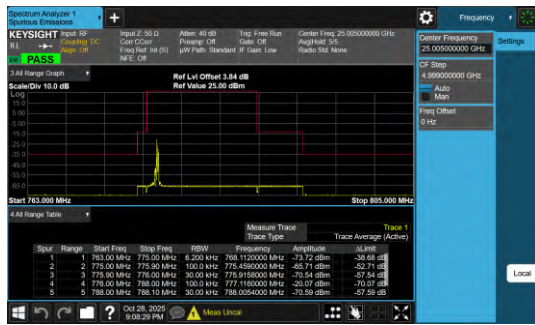
Band13-0.18-BPSK-23181-PASS
