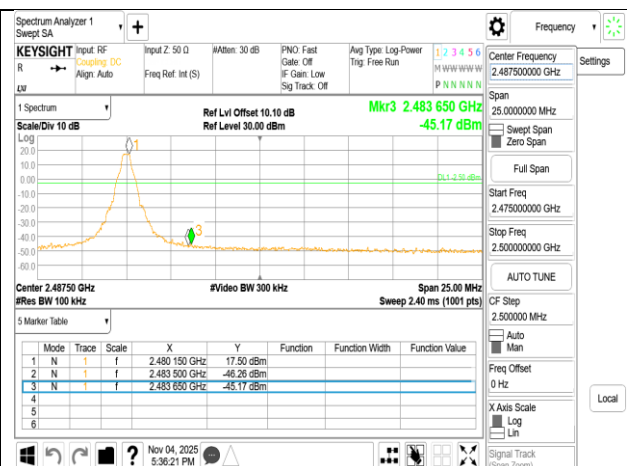
Band Edge GFSK 1M DH5 2480MHz
