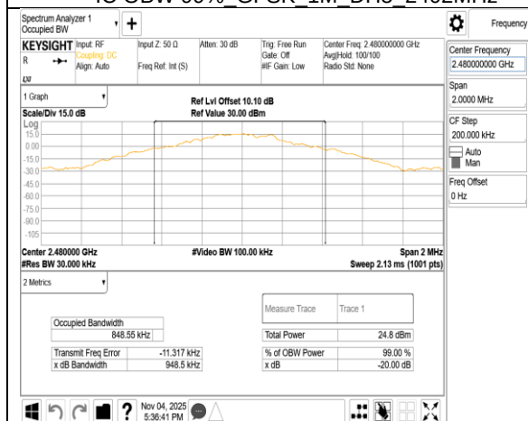
IC OBW 99% GFSK 1M DH5 2480MHz
