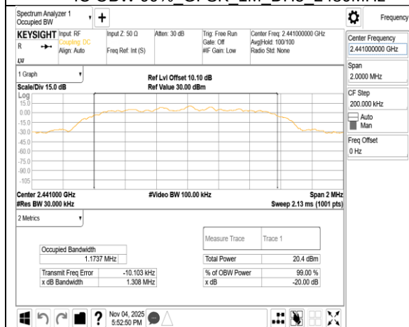
IC OBW 99% \pi/4 DQPSK 2M DH5 2441MHz
