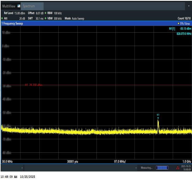
11G-Ant1-2462-30~1000-PASS
