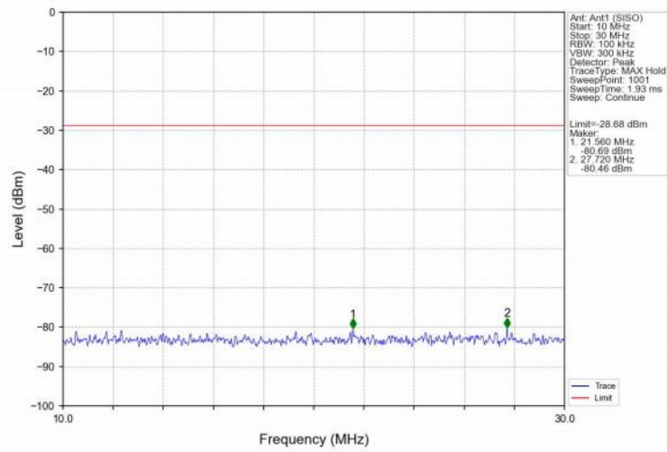
802.11n(HT20)_HCH_2462MHz_Ant1 (SISO)_NTNV
