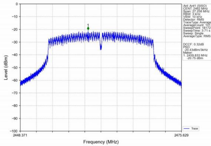
802.11n(HT20)_HCH_2462MHz_Ant1 (SISO)_NTNV
