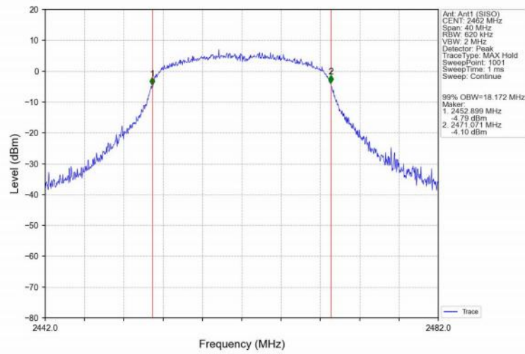
802.11n(HT20)_HCH_2462MHz_Ant1 (SISO)_NTNV
