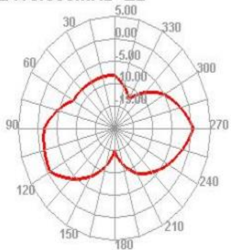
2460.000MHz E2
