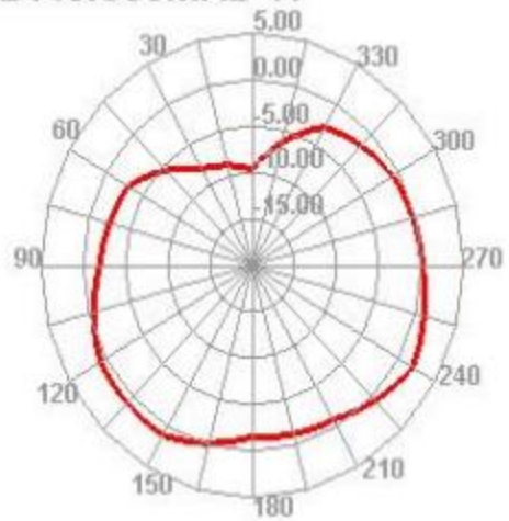
2440.000MHz H
