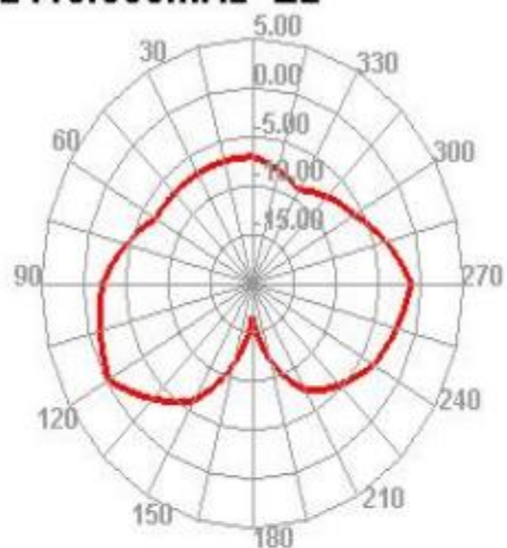
2410.000MHz E2
