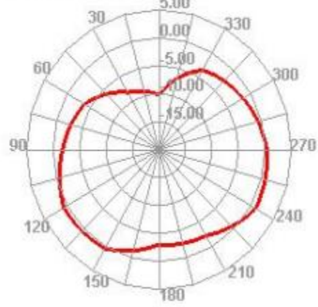
2470.000MHz H
