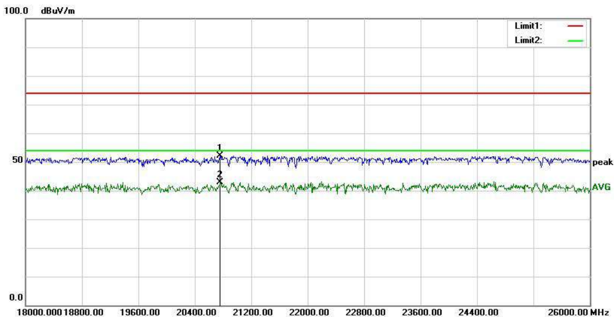
RSE-L-18GHz-26GHz-H
