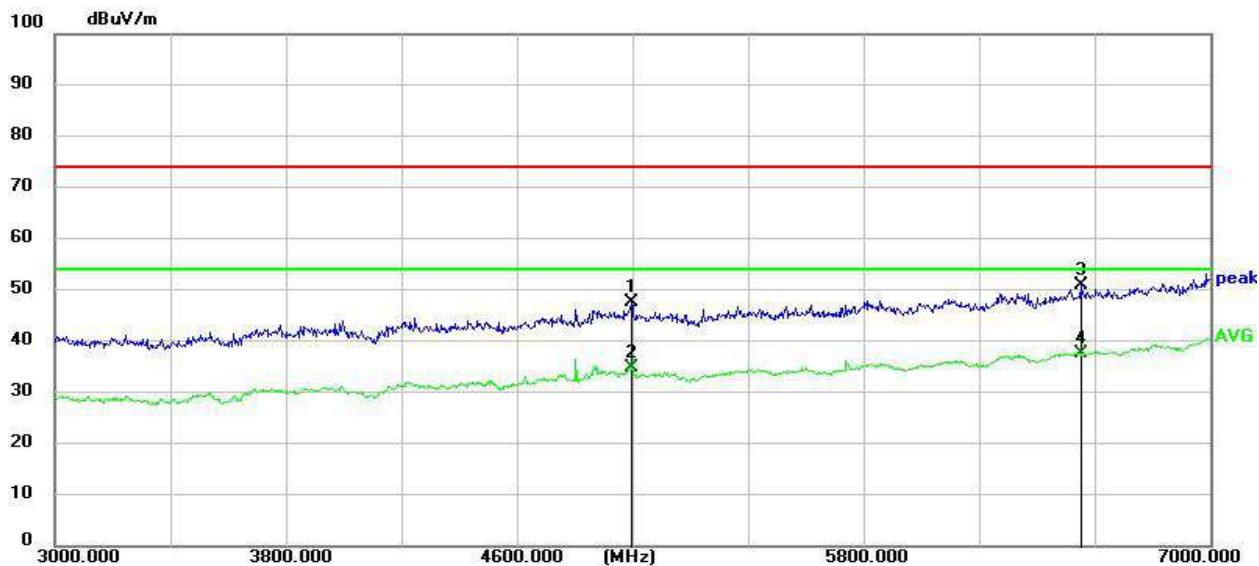
RSE-L-3GHz-7GHz-V
