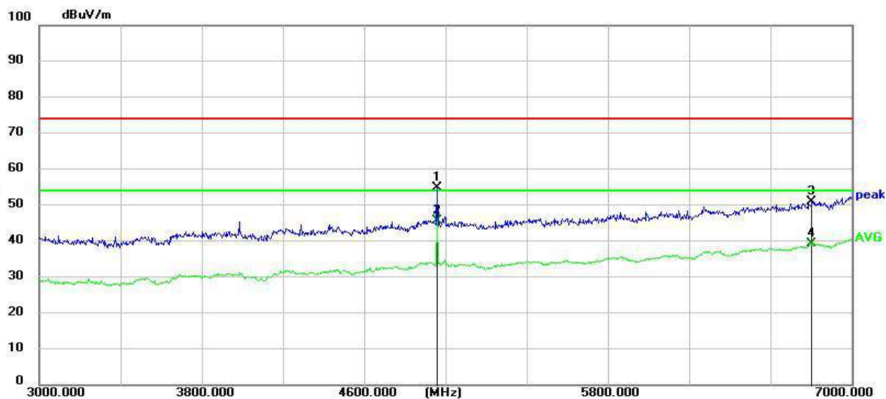
RSE-H-3GHz-7GHz-V
