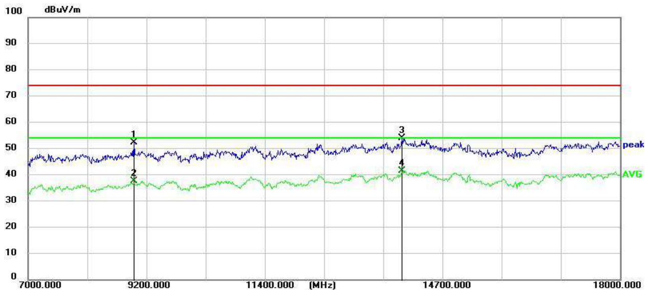
RSE-H-7GHz-18GHz-V
