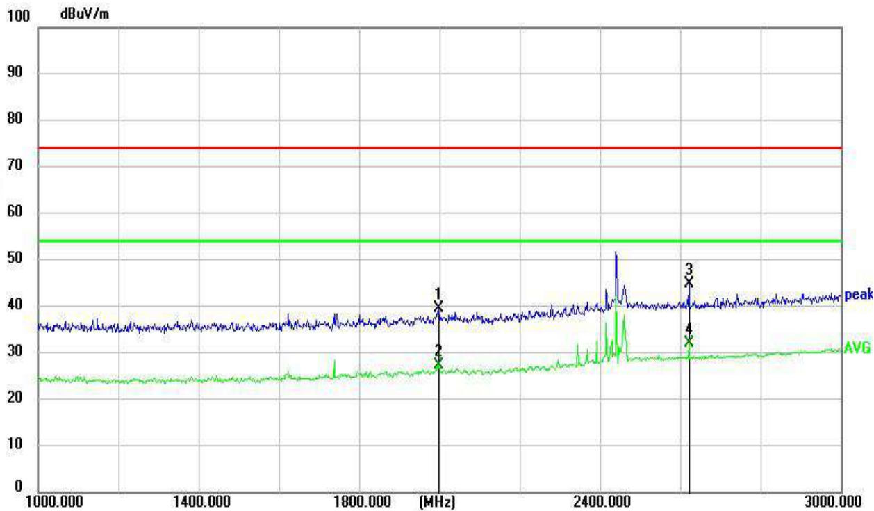
RSE-M-1GHz-3GHz-V
