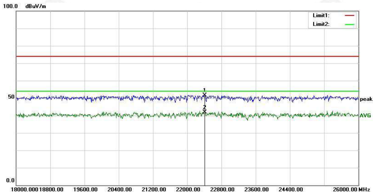
RSE-M-18GHz-26GHz-V
