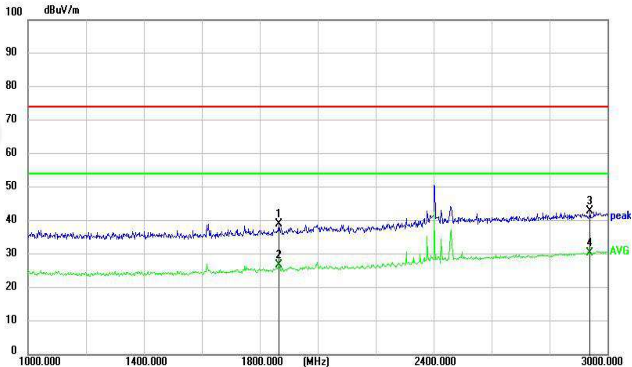
RSE-L-1GHz-3GHz-V
