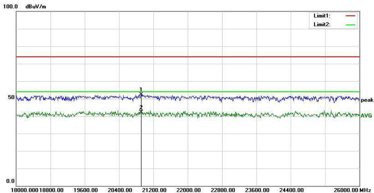
RSE-L-18GHz-26GHz-V
