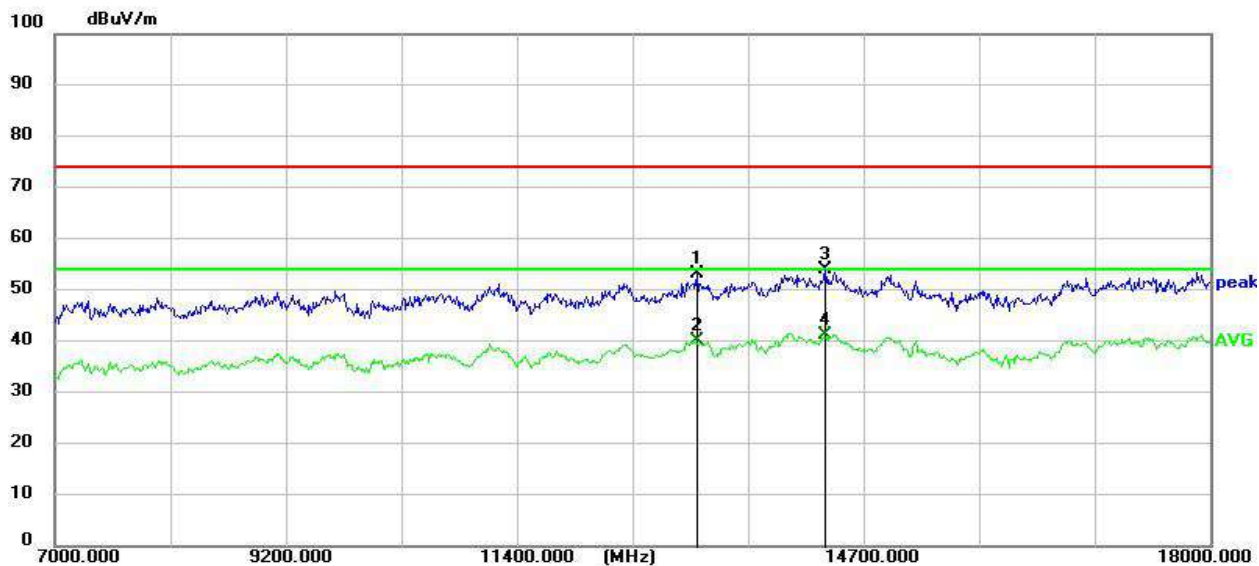
RSE-M-7GHz-18GHz-V
