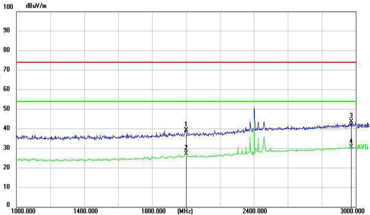
RSE-L-1GHz-3GHz-V
