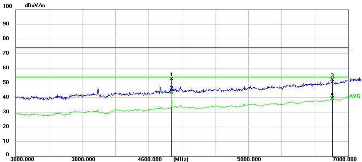
RSE-M-3GHz-7GHz-V
