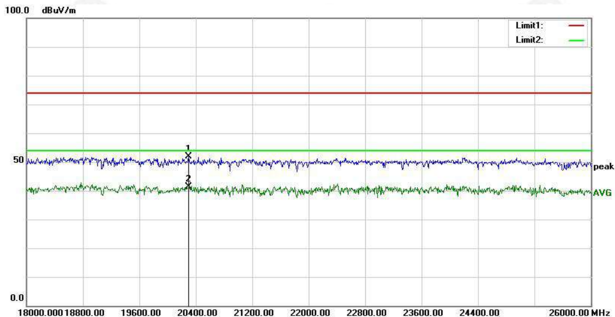
RSE-H-18GHz-26GHz-V
