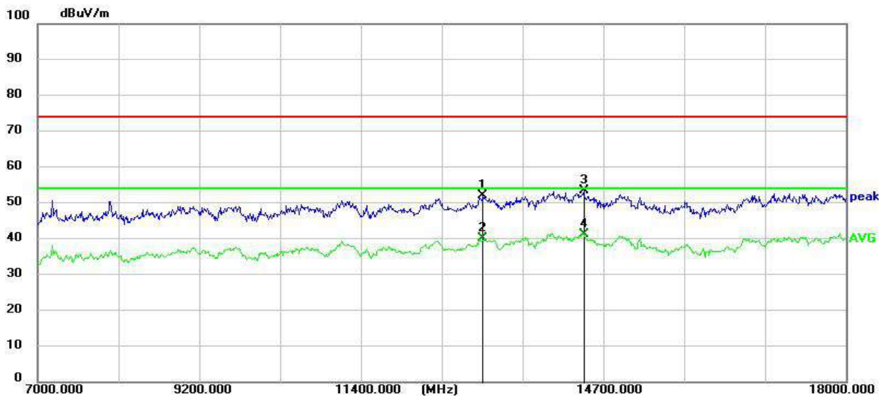
RSE-L-7GHz-18GHz-V
