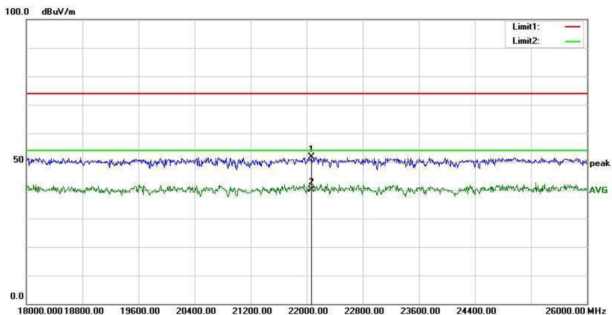
RSE-H-18GHz-26GHz-V
