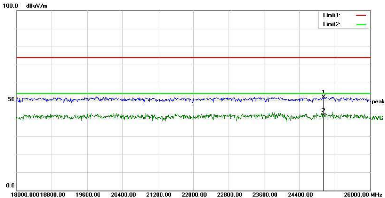
RSE-L-18GHz-26GHz-V
