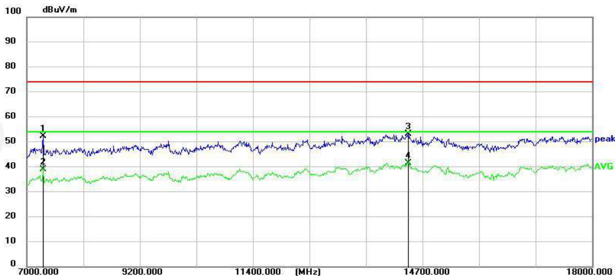
RSE-M-7GHz-18GHz-H
