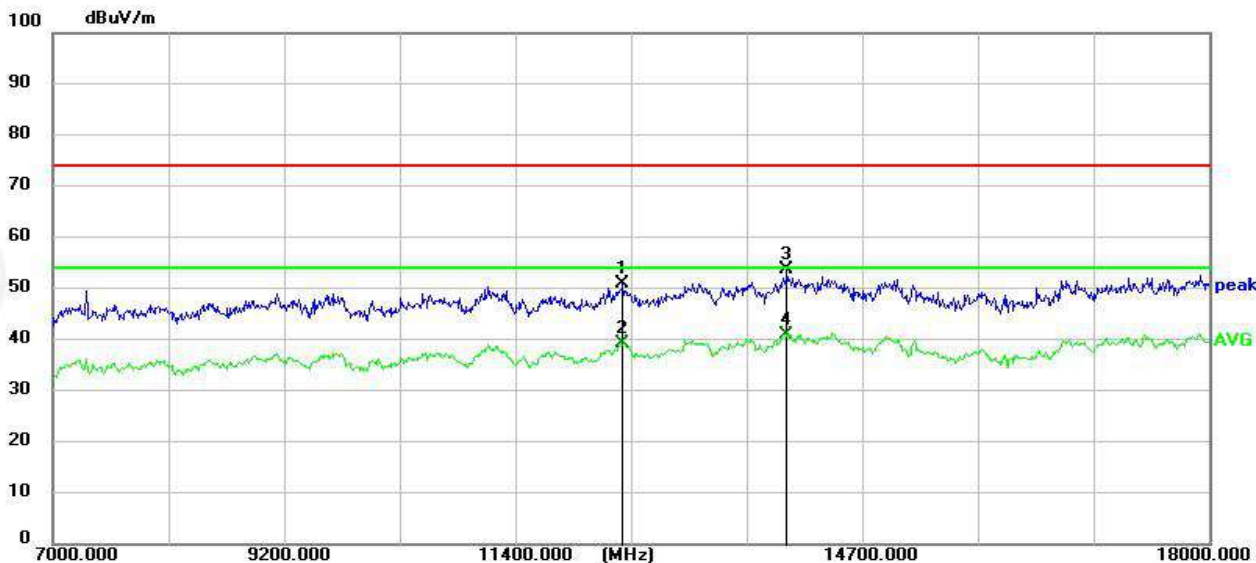
RSE-M-7GHz-18GHz-H
