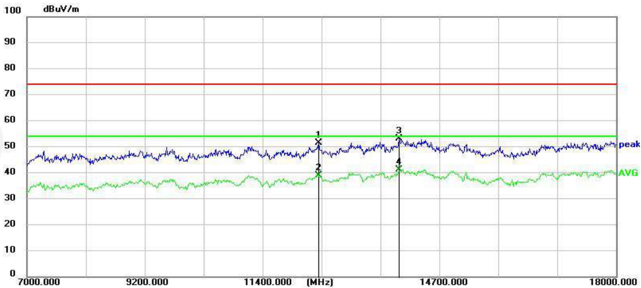
RSE-M-7GHz-18GHz-H
