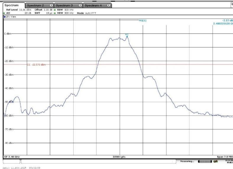
LE 1M_Ant1_2480_Band Edge
