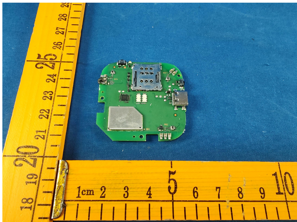
Wi-Fi ANT
