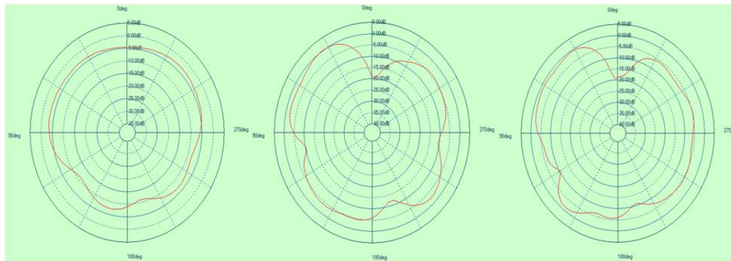
2350MHz (Phi0/Phi90/Theta90)
