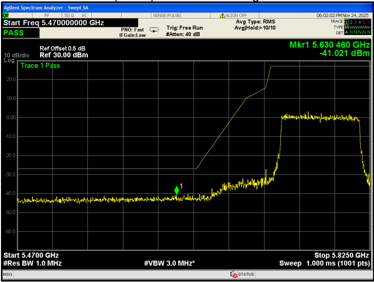
802.11ax(HE80) U-NII-3 Band edge-left side
