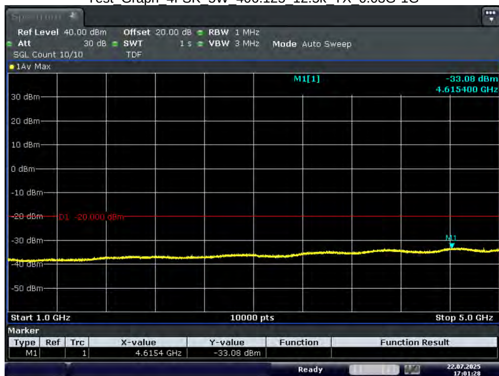
Test_Graph_4FSK_5W_406.125_12.5k_TX_1G-5G
