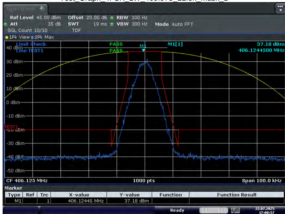
Test_Graph_4FSK_5W_406.125_12.5k_Mask_D
