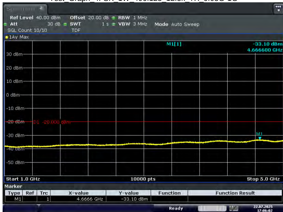
Test_Graph_4FSK_1W_406.125_12.5k_TX_1G-5G
