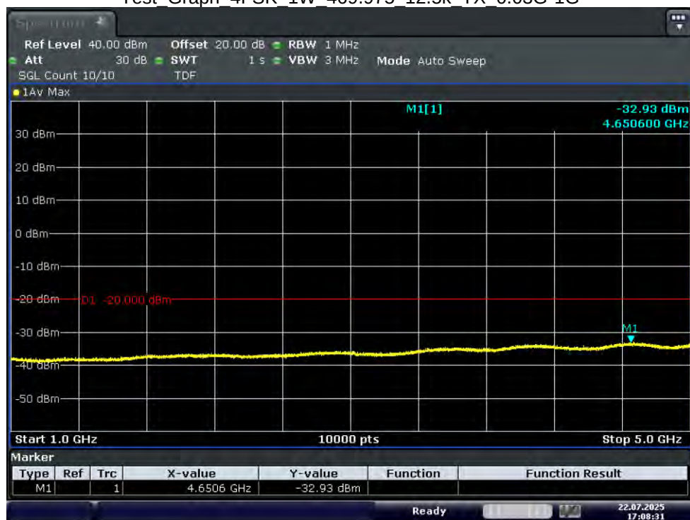
Test_Graph_4FSK_1W_469.975_12.5k_TX_1G-5G
