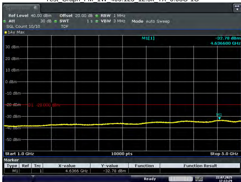
Test_Graph_FM_1W_406.125_12.5k_TX_1G-5G
