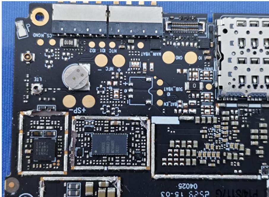
Bluetooth/WIFI/WWAN/GPS Antenna
