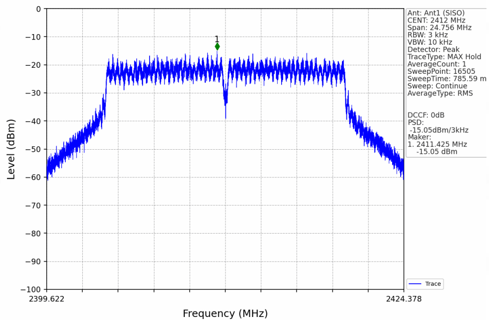
802.11g_LCH_2412MHz_Ant1 (SISO)_NTNV
