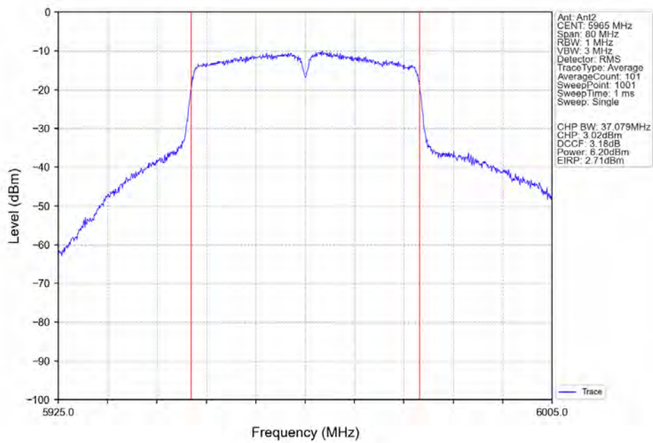
802.11ac(VHT40) LCH 5965MHz Ant2 NTN
