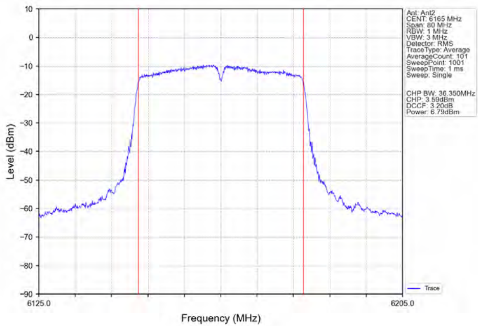
802.11ac(VHT40) MCH 6165MHz Ant2 NTNV
