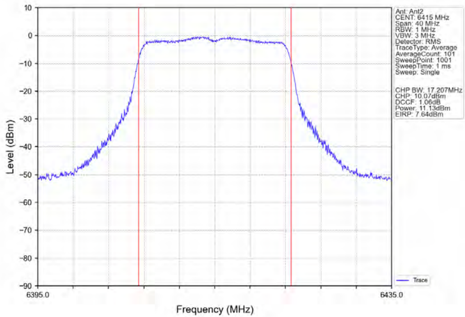
802.11a HCH 6415MHz Ant2 NTN
