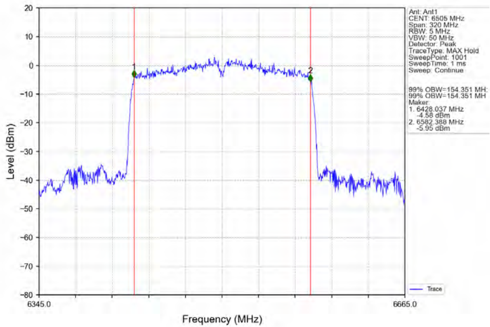
802.11ac(VHT160) HCH 6505MHz Ant1 NTN
