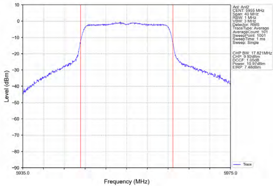
802.11a LCH 5955MHz Ant2 NTN
