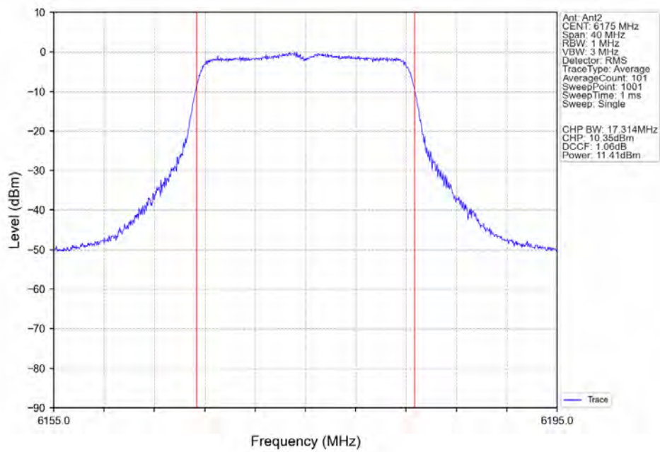
802.11a MCH 6175MHz Ant2 NTNV
