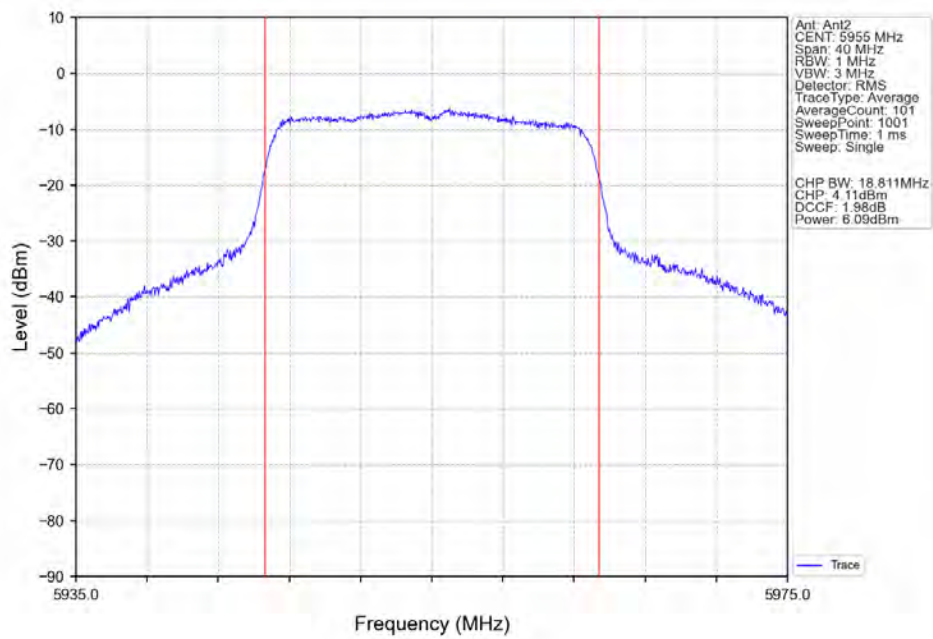
802.11ac(VHT20) LCH 5955MHz Ant2 NTNV
