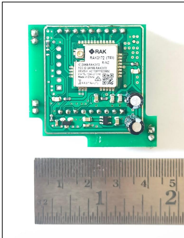
Photo 15: ANSI EM Addon Module card front view
