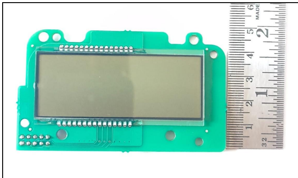
Photo 10: ANSI EM Display Card front view
