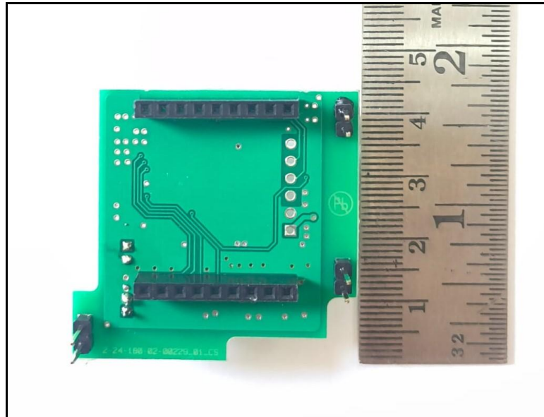
Photo 16: ANSI EM Addon Module card rare view
