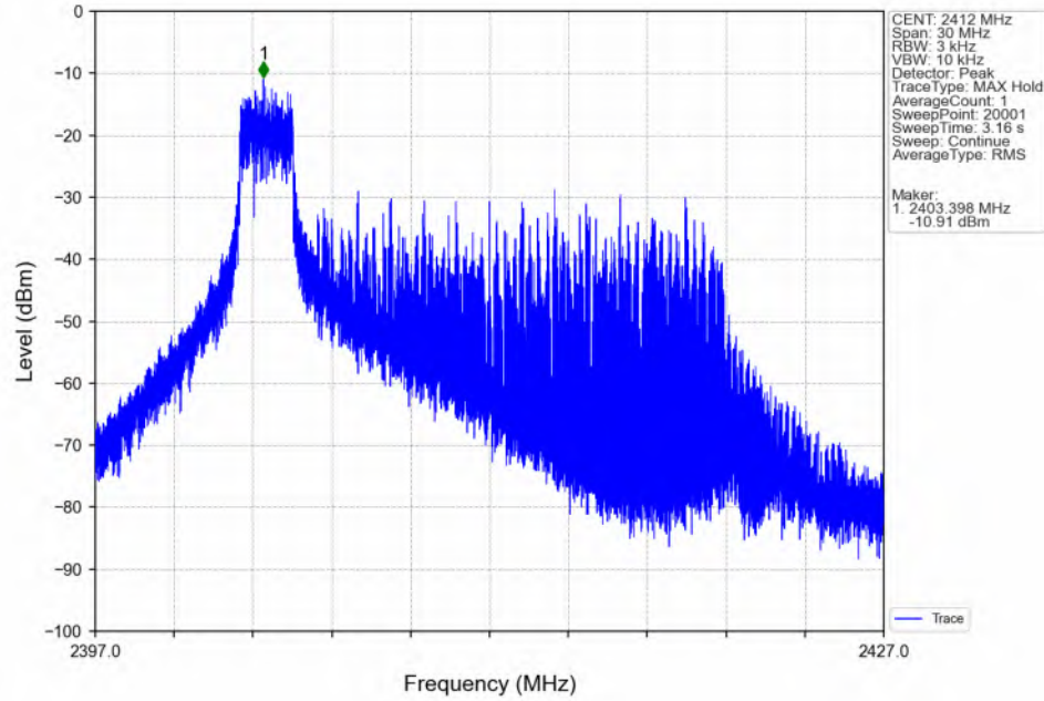
802.11ax(HEW20)_LCH_2412MHz_RU26_Left_Ant7(MIMO)_NTNV
