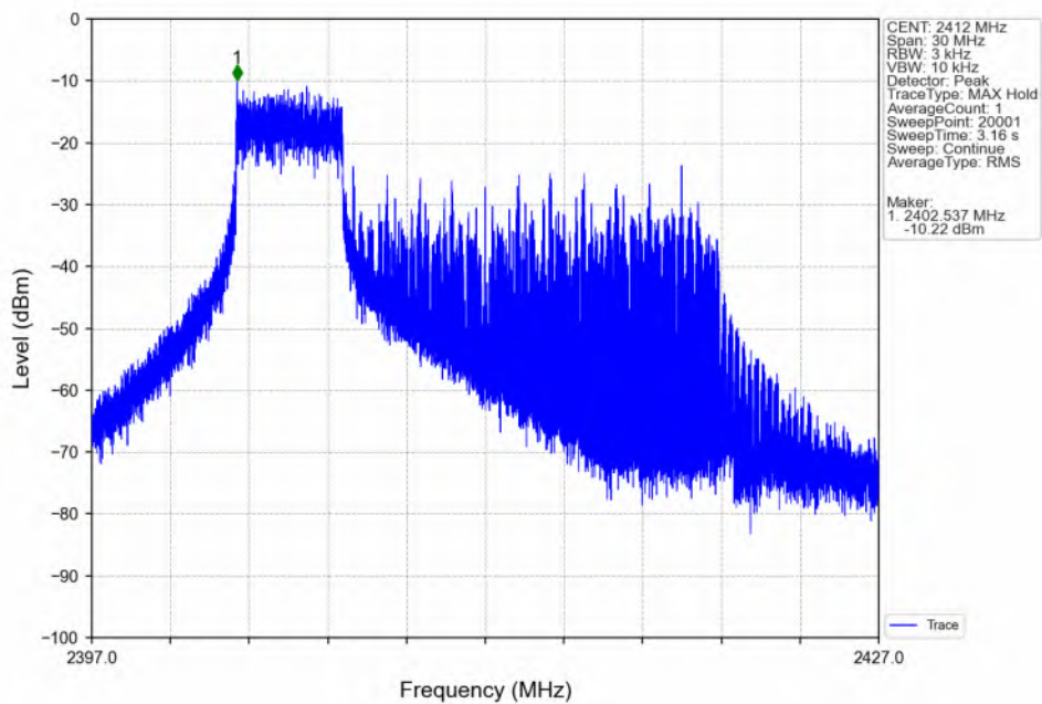
802.11ax(HEW20)_LCH_2412MHz_RU52_Left_Ant6(MIMO)_NTNV
