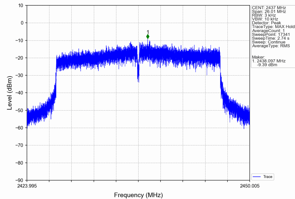
802.11ax(HEW20) MCH 2437MHz SU / Ant6 (MIMO) NTN
