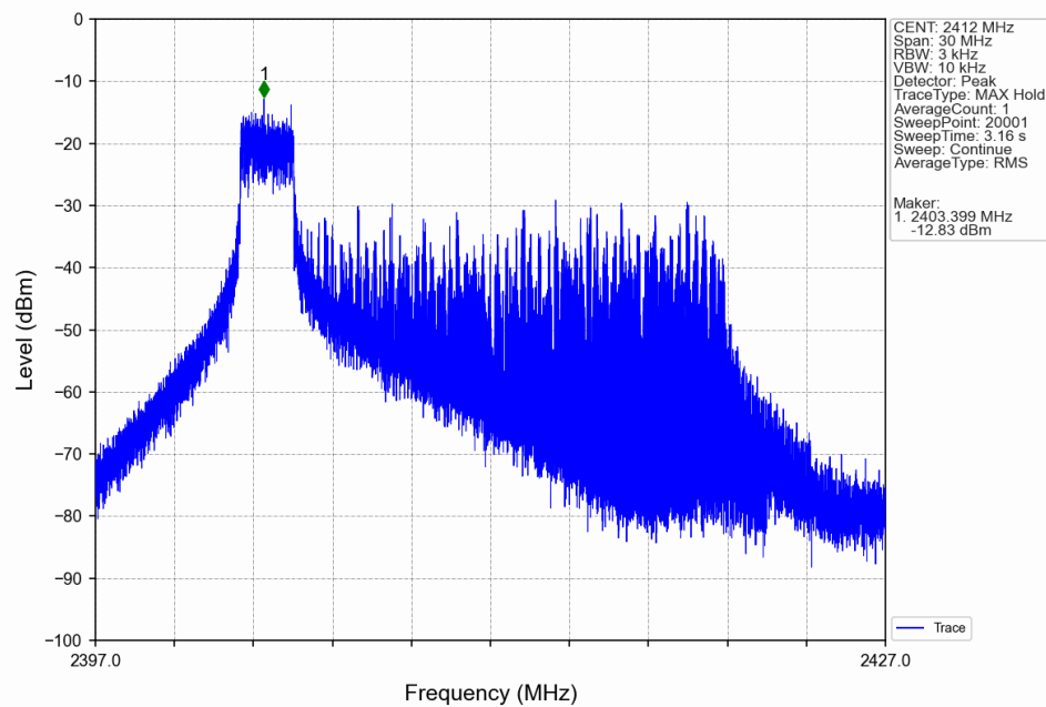
802.11ax(HEW20)_LCH_2412MHz_RU26_Left_Ant7(MIMO)_NTNV
