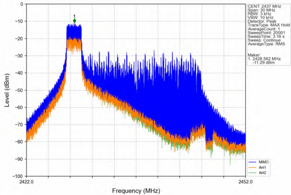
802.11ax(HEW20)_MCH_2437MHz_RU52_Left_Ant6(MIMO)_NTNV
