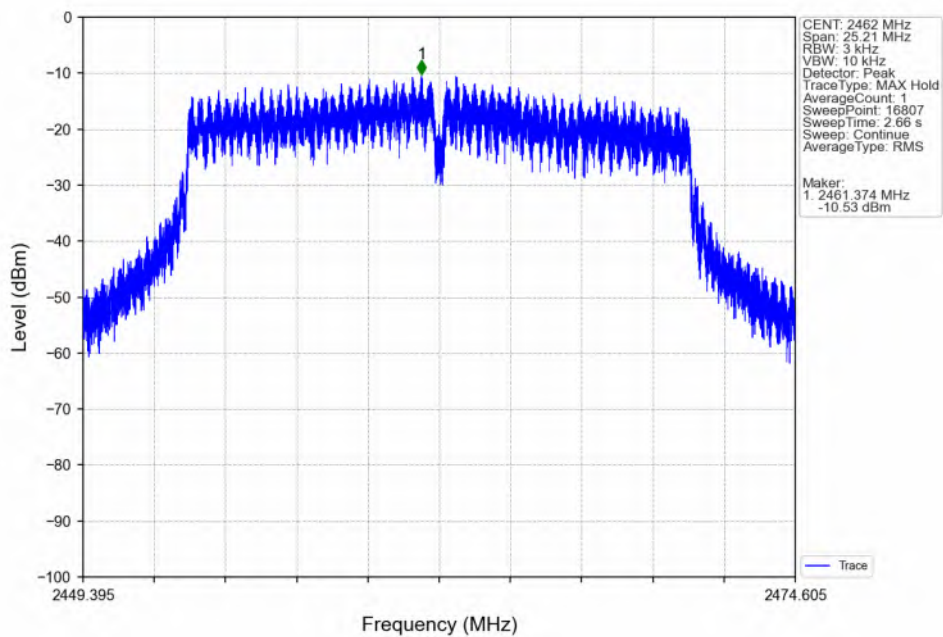
802.11n(HT20) HCH 2462MHz_Ant7 (MIMO) NTN
