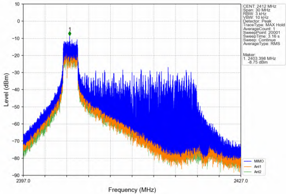
802.11ax(HEW20)_LCH_2412MHz_RU52_Left_Ant6(MIMO)_NTNV
