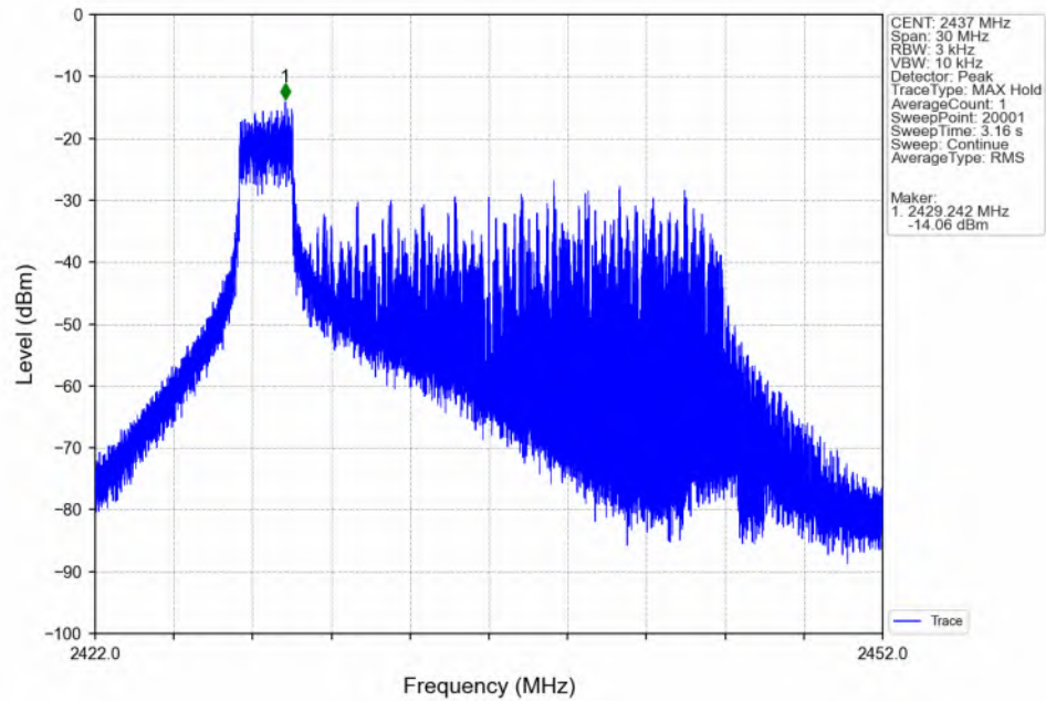
802.11ax(HEW20) MCH_2437MHz RU26_Left_Ant7 (MIMO) NTNv
