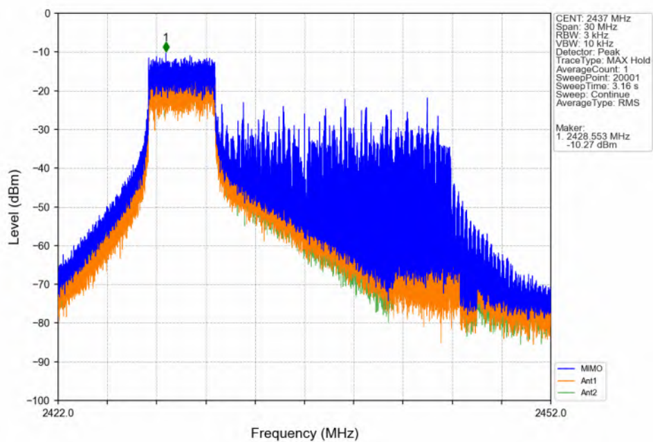
802.11ax(HEW20) MCH_2437MHz RU52 Left MIMO NTN
