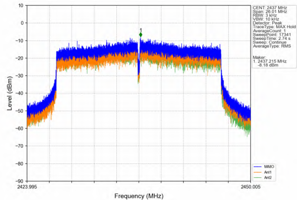
802.11ax(HEW20) MCH 2437MHz SU / MIMO NTN
