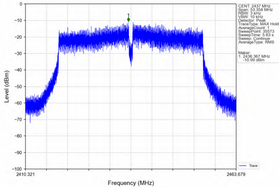
802.11n(HT40) MCH_2437MHz_Ant7 (MIMO) NTN
