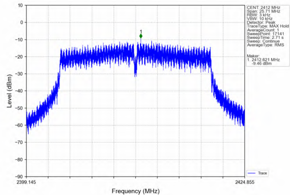
802.11n(HT20) LCH 2412MHz_Ant7 (MIMO) NTN
