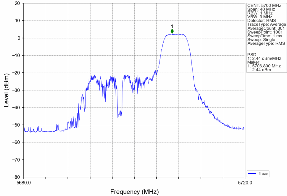
802.11ax(HEW20) HCH_5700MHz RU52 Right_Ant7 NTN
