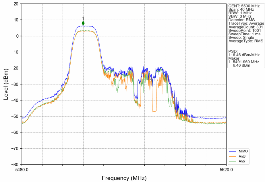
802.11ax(HEW20) LCH_5500MHz RU106 Left Ant6 NTN
