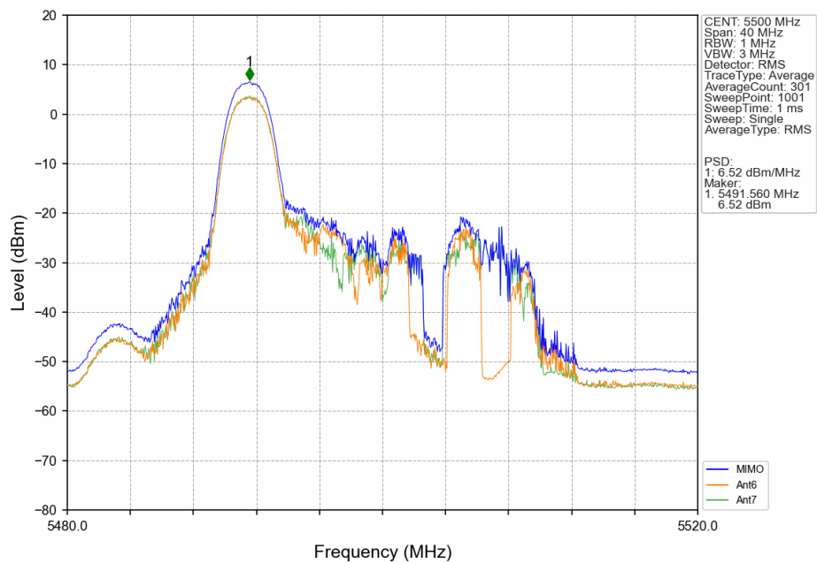
802.11ax(HEW20) LCH_5500MHz_RU26_Left_MIMO_NTNV
