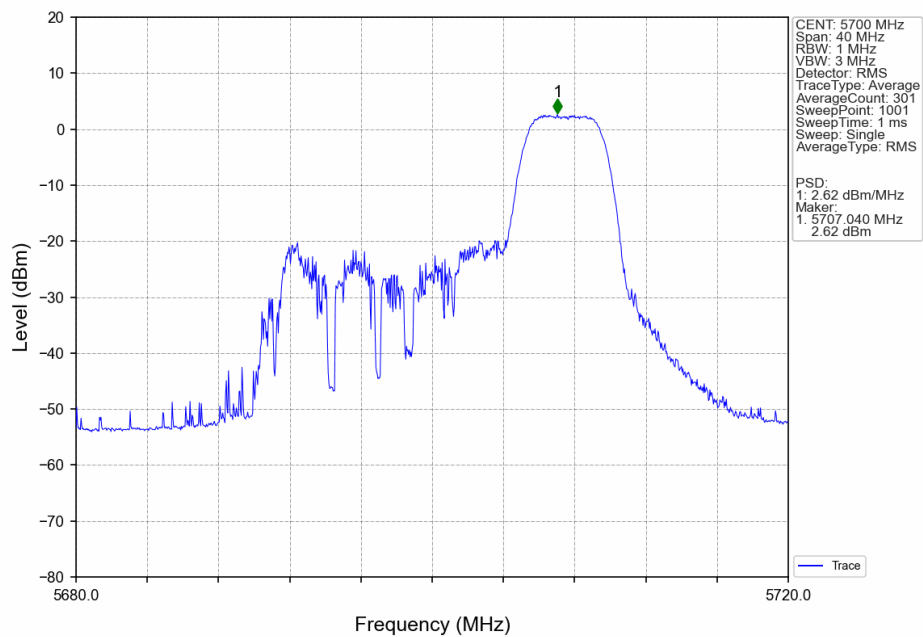
802.11ax(HEW20) HCH_5700MHz RU52 Right_Ant7 NTN
