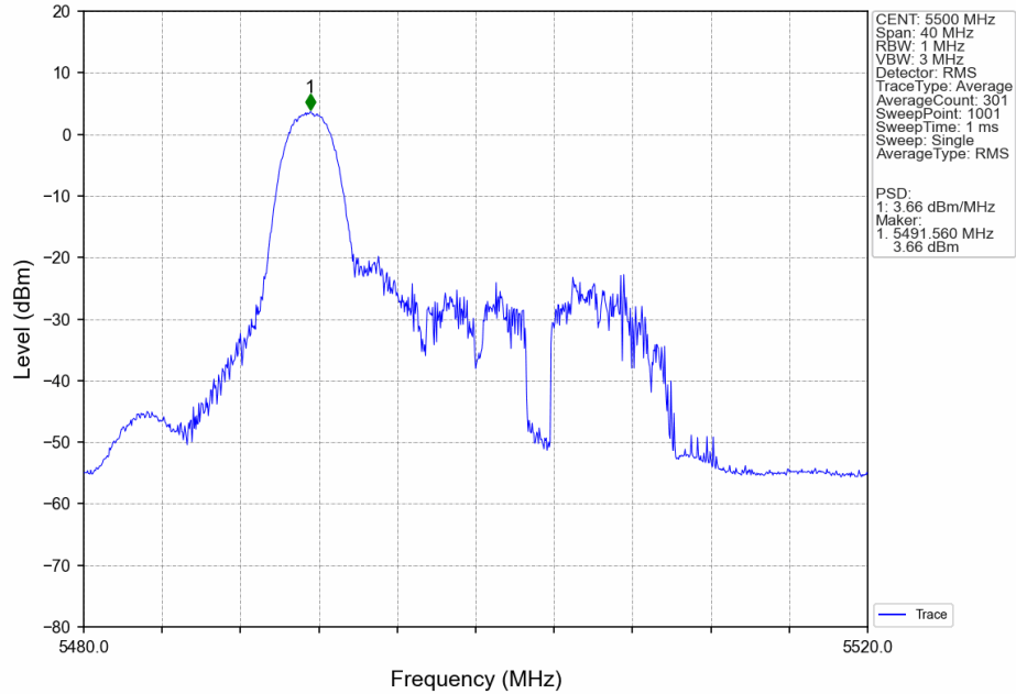
802.11ax(HEW20) LCH_5500MHz_RU26_Left_MIMO_NTNV
