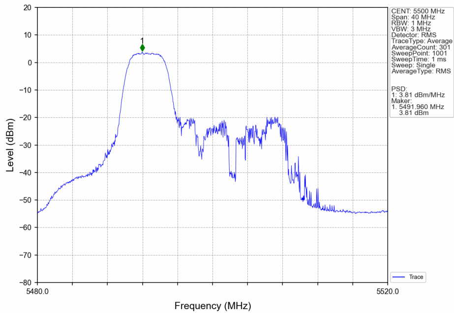
802.11ax(HEW20) LCH 5500MHz RU52 Left Ant7 NTN
