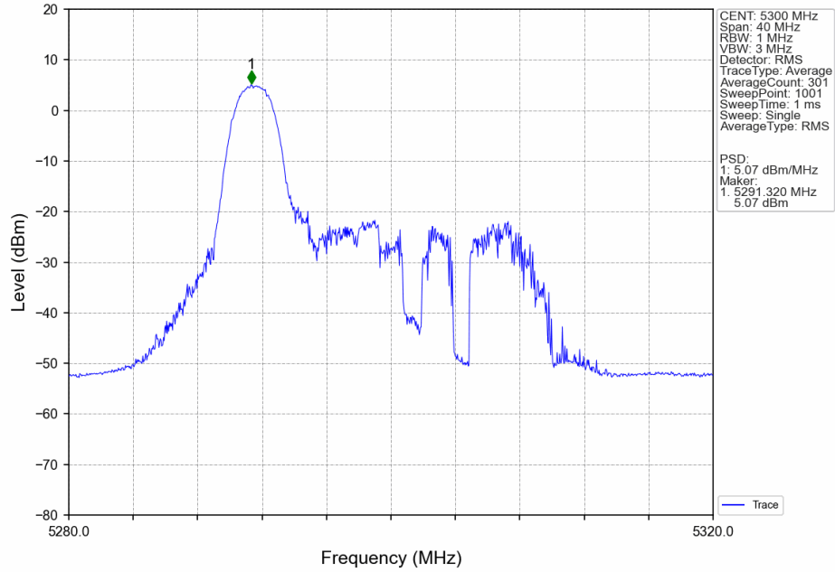
802.11ax(HEW20) MCH 5300MHz RU26 Left MIMO NTN
