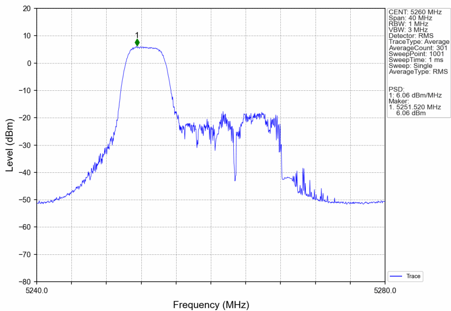
802.11ax(HEW20) LCH 5260MHz RU52 Left Ant7 NTN
