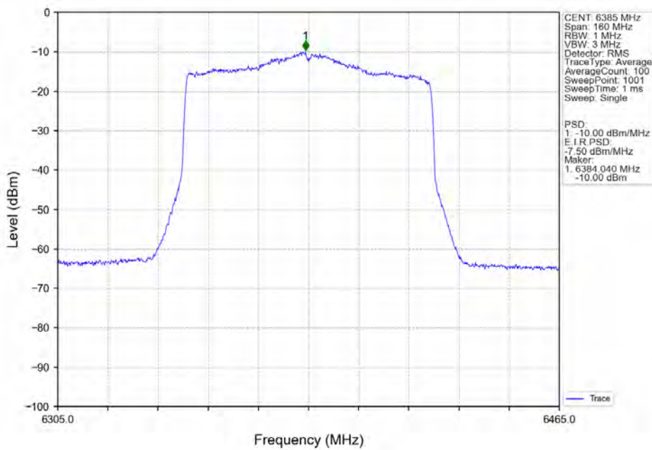
802.11ax(HEW80) HCH_6385MHz_SU / Ant7 NTN
