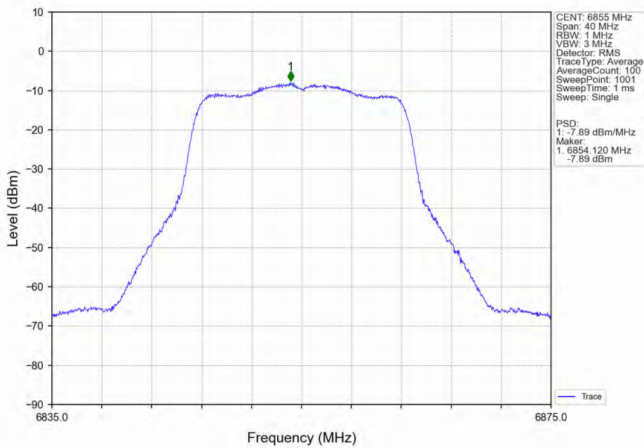
802.11a_HCH_6855MHz_Ant7_NTNV
