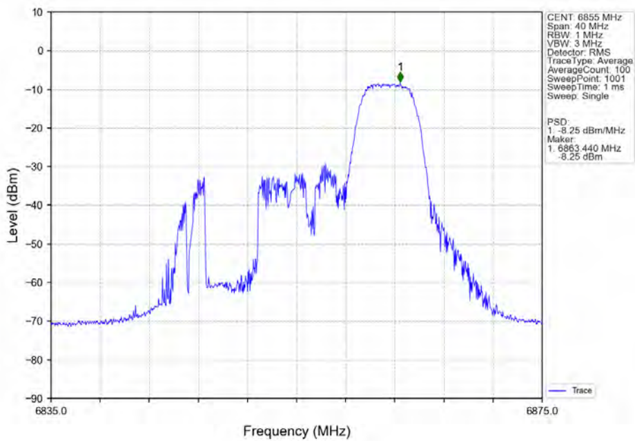
802.11ax(HEW20)_HCH_6855MHz_RU52_Right_Ant7_NTNV
