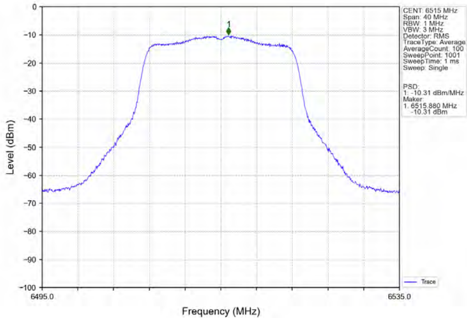
802.11a_HCH_6515MHz_Ant7_NTNV
