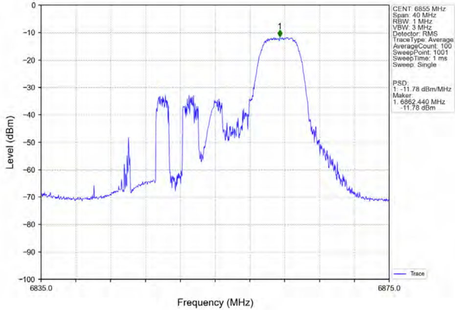
802.11ax(HEW20)_HCH_6855MHz_RU52_Right_Ant7_NTNV
