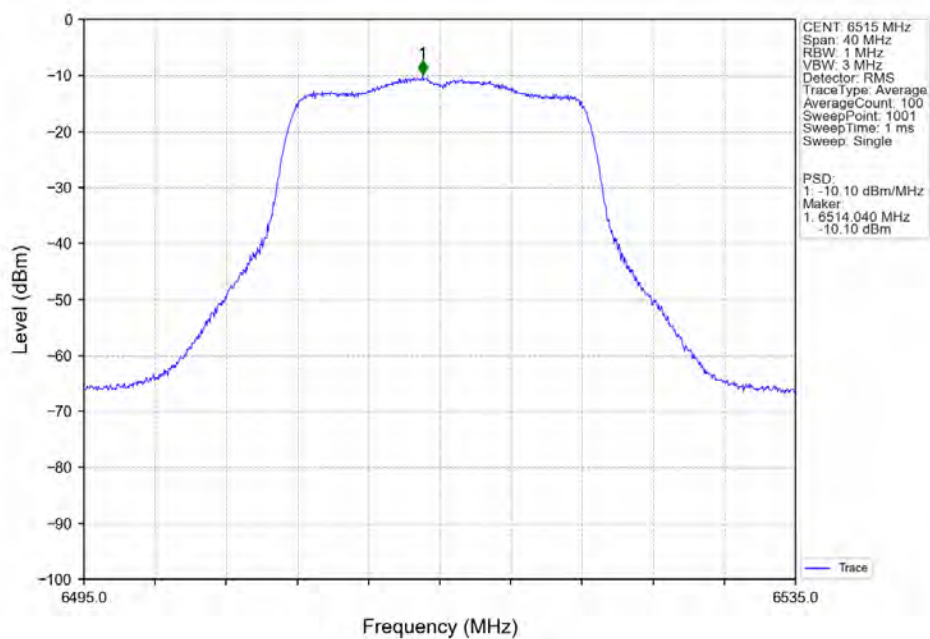
802.11a_HCH_6515MHz_Ant7_NTNV
