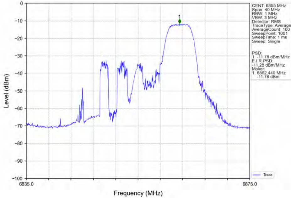
802.11ax(HEW20)_HCH_6855MHz_RU52_Right_Ant7_NTNV
