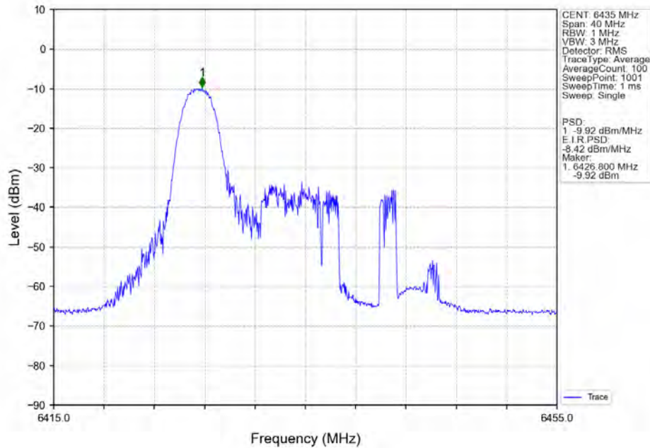
802.11ax(HEW20) LCH 6435MHz RU26 Left MIMO NTN
