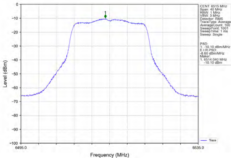
802.11a_HCH_6515MHz_Ant7_NTNV
