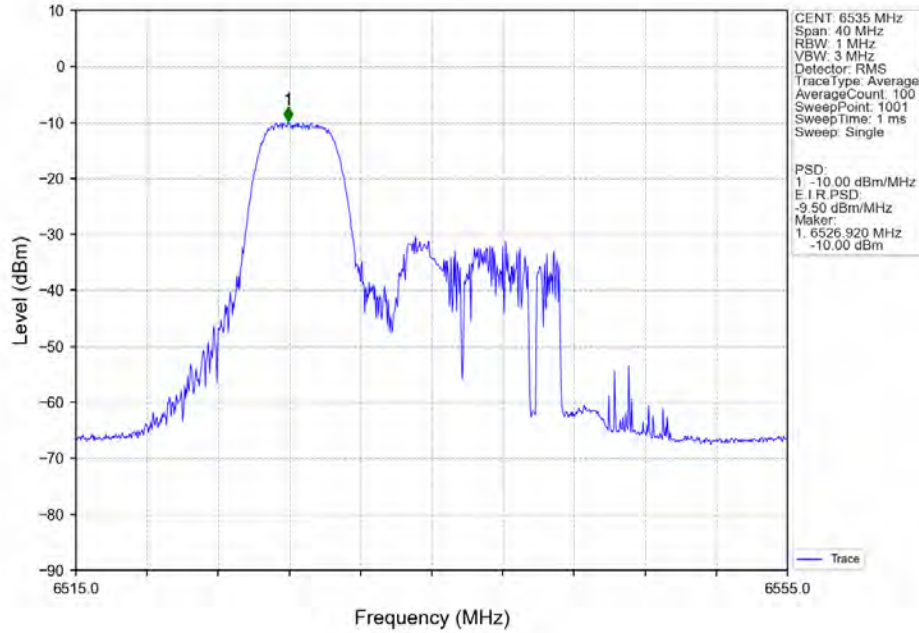
802.11ax(HEW20) LCH 6535MHz RU52 Left Ant7 NTN
