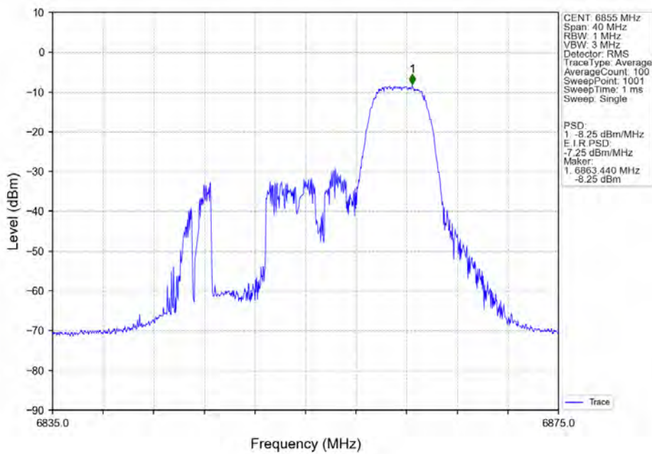
802.11ax(HEW20)_HCH_6855MHz_RU52_Right_Ant7_NTNV
