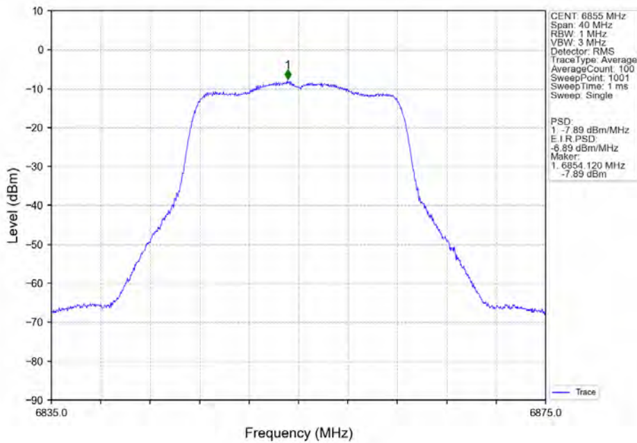
802.11a_HCH_6855MHz_Ant7_NTNV
