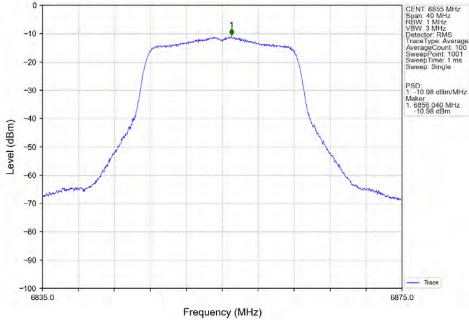
802.11a_HCH_6855MHz_Ant7_NTNV
