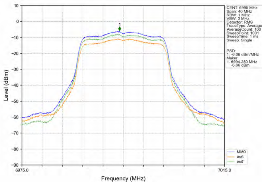
802.11a MCH 6995MHz MIMO NTN
