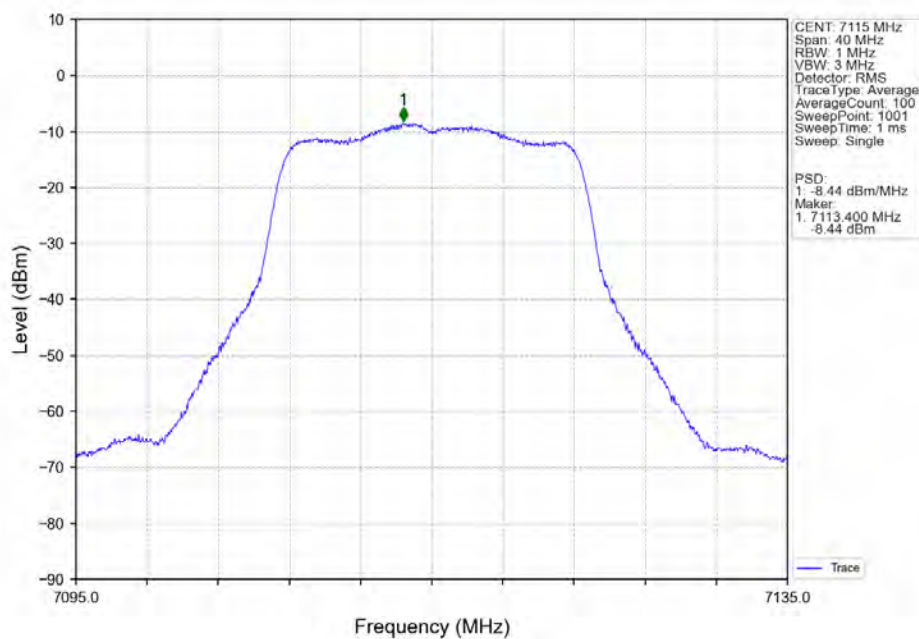
802.11a_HCH_7115MHz_Ant7_NTNV
