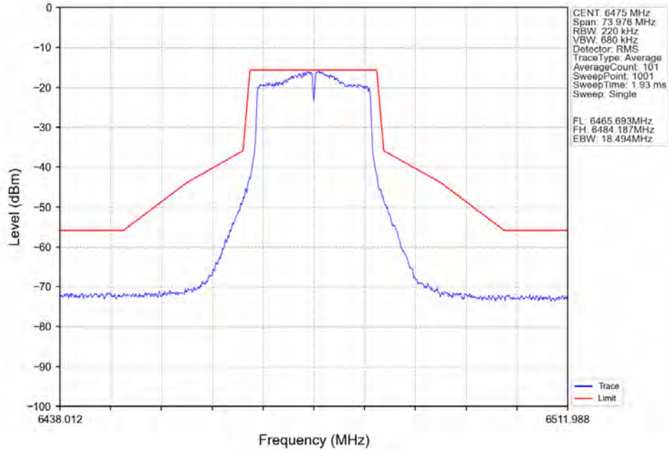
802.11a_MCH_6475MHz_Ant7_NTNV
