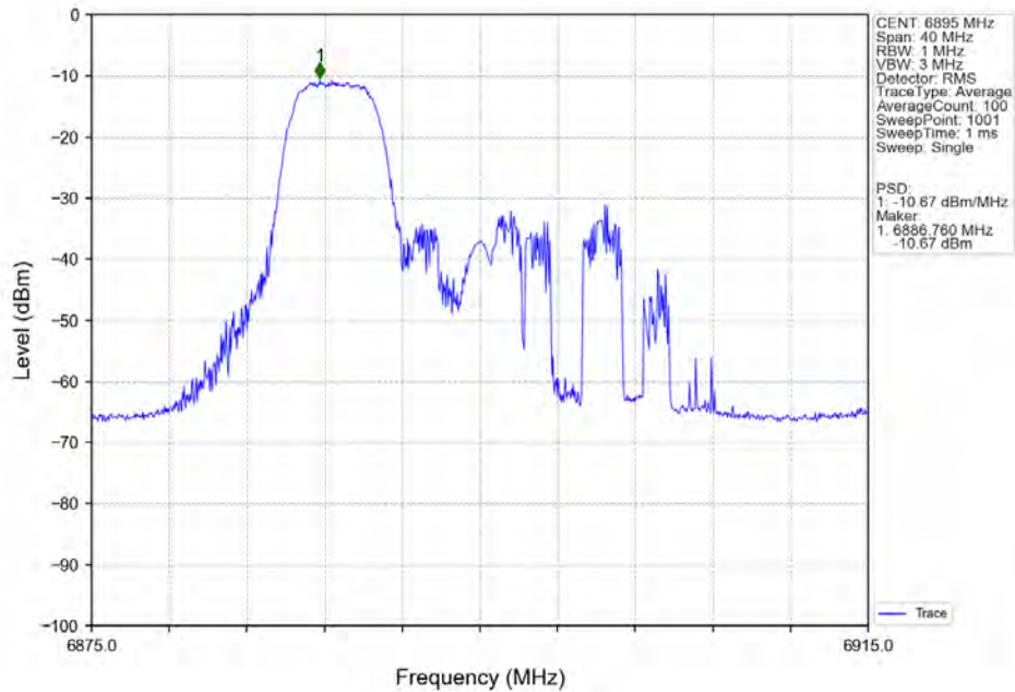
802.11ax(HEW20) LCH 6895MHz RU52 Left Ant7 NTN
