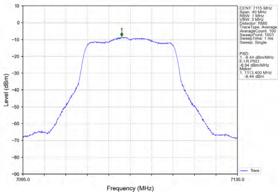
802.11a_HCH_7115MHz_Ant7_NTNV
