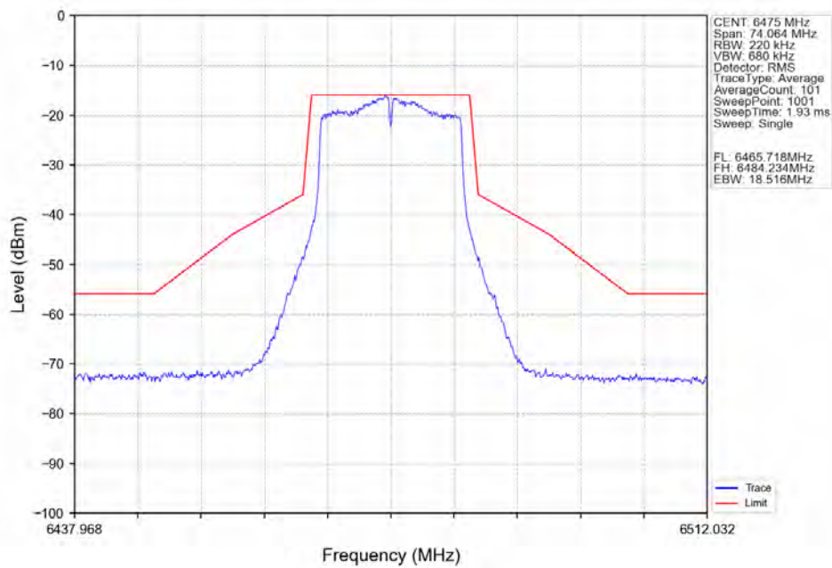
802.11a_MCH_6475MHz_Ant7_NTNV
