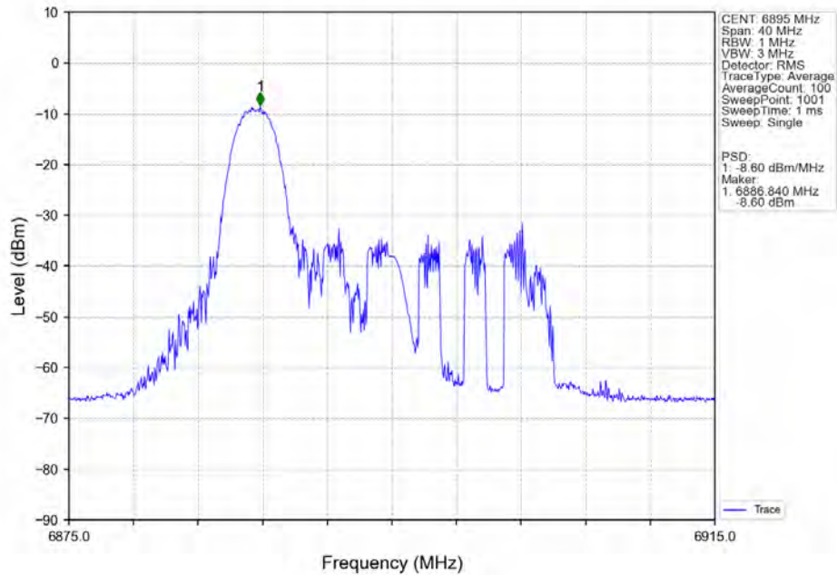
802.11ax(HEW20) LCH_6895MHz_RU26_Left_MIMO_NTNV
