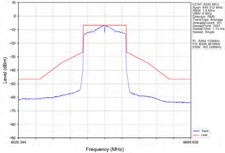
802.11ax(HEW160) HCH 6345MHz SU / Ant7 NTN
