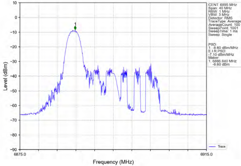
802.11ax(HEW20) LCH_6895MHz_RU26_Left_MIMO_NTNV
