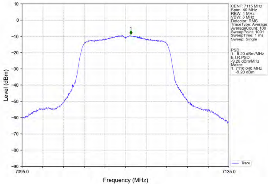
802.11a_HCH_7115MHz_Ant7_NTNV
