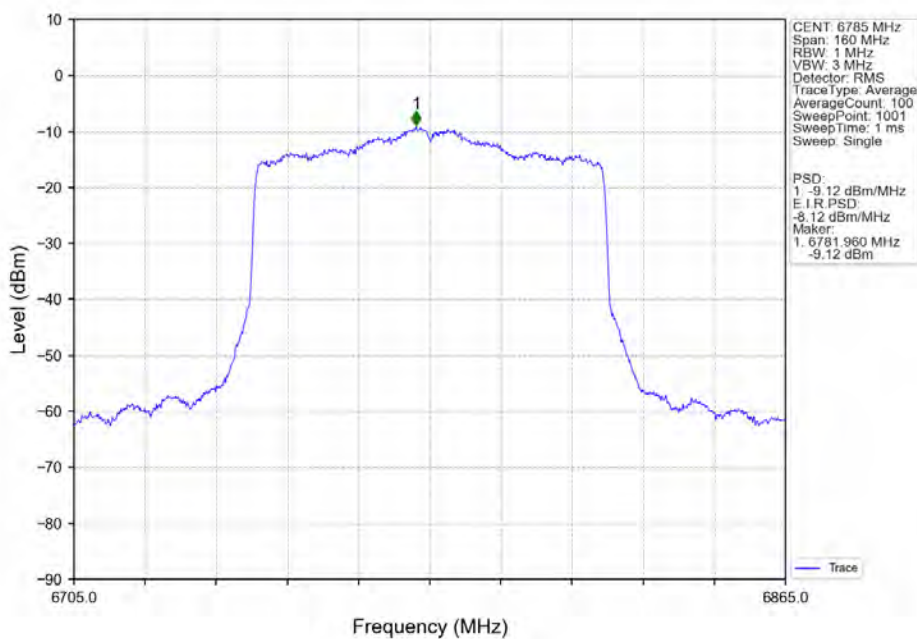
802.11ax(HEW80) HCH_6785MHz_SU / Ant7 NTN
