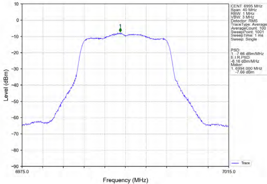
802.11a_MCH_6995MHz_MIMO_NTNV
