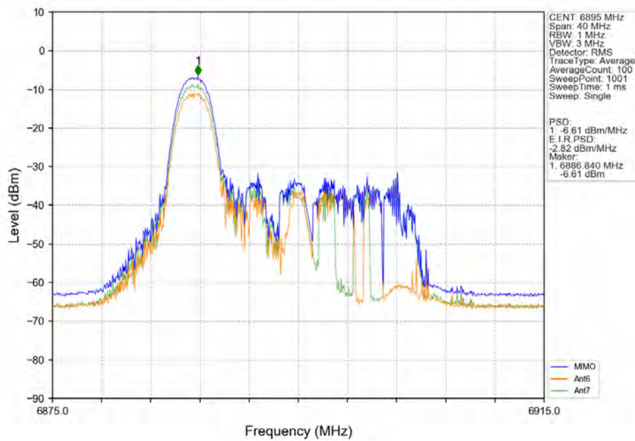
802.11ax(HEW20) LCH_6895MHz_RU26_Left_MIMO_NTNV
