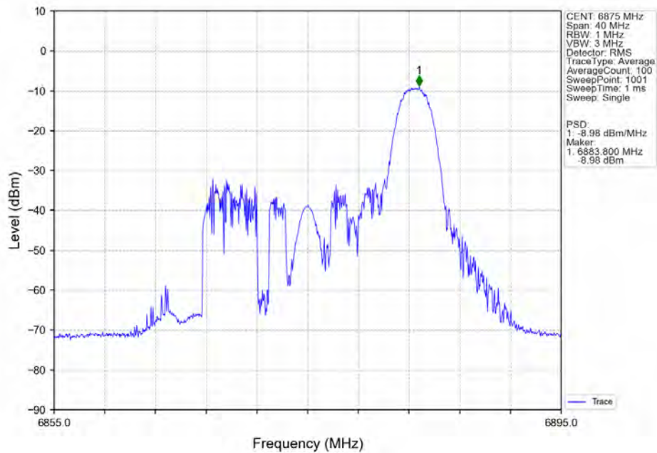
802.11ax(HEW20) HCH 6875MHz RU26 Right MIMO NTN
