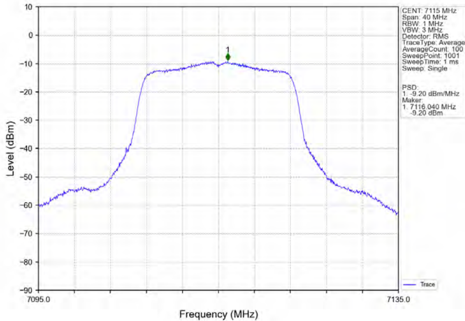
802.11a_HCH_7115MHz_Ant7_NTNV
