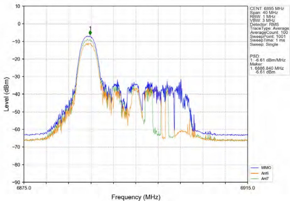
802.11ax(HEW20) LCH_6895MHz_RU26_Left_MIMO_NTNV
