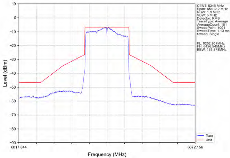
802.11ax(HEW160) HCH 6345MHz SU / Ant7 NTN
