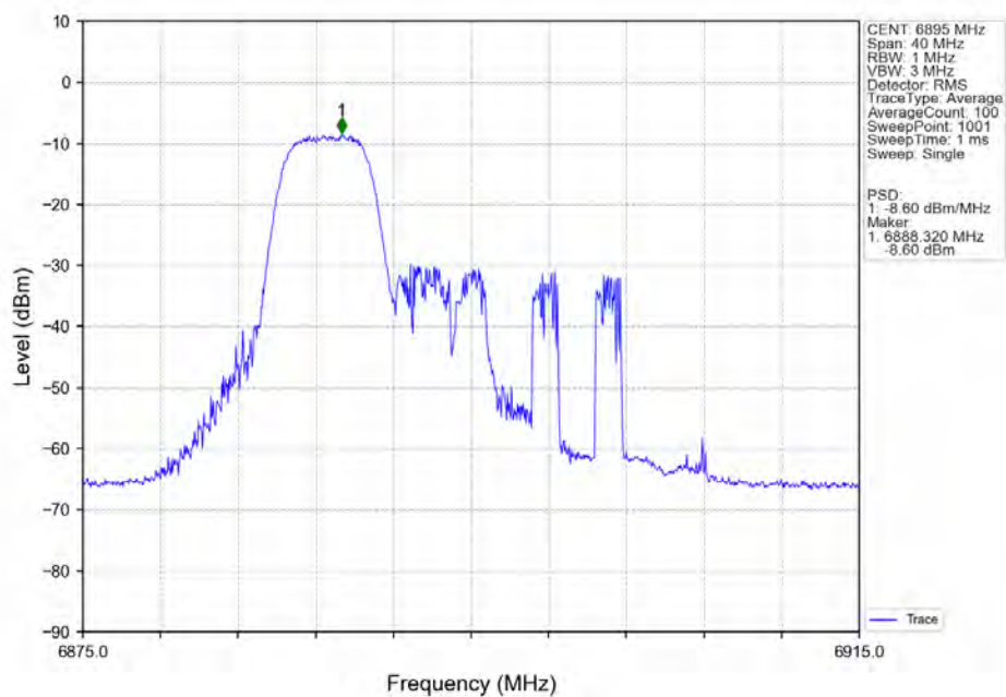
802.11ax(HEW20) LCH 6895MHz RU52 Left Ant7 NTN
