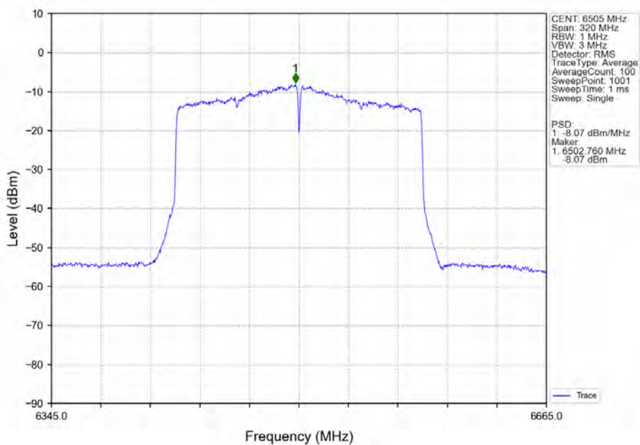
802.11ax(HEW160) HCH 6505MHz_SU / _Ant7_NTNV
