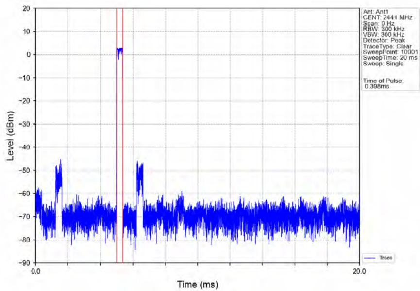
GFSK_DH1_HOPP_Ant1_NTNV
