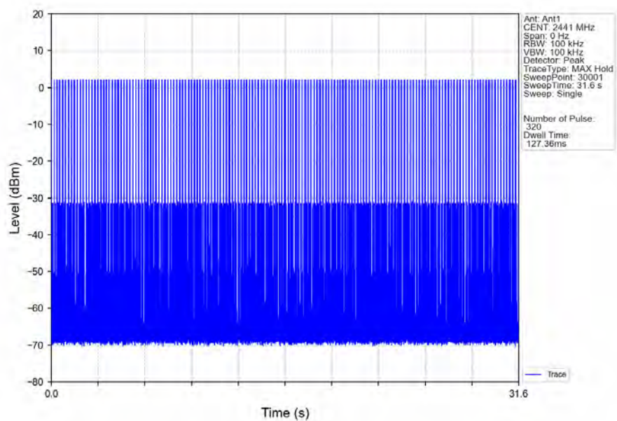
GFSK_DH1_HOPP_Ant1_NTNV
