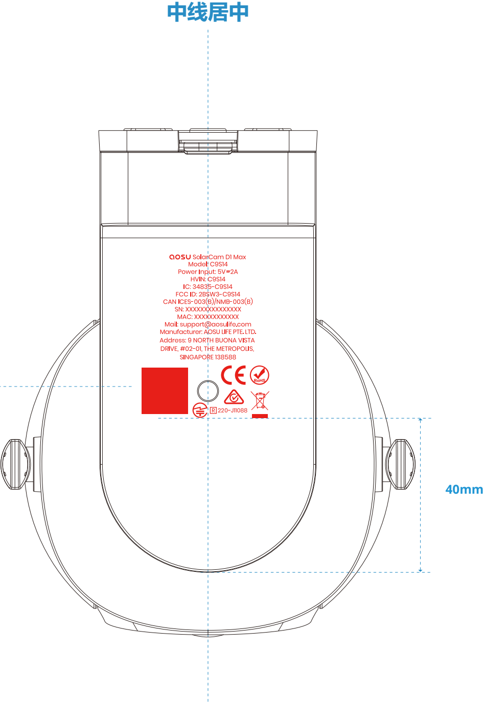
产品顶部俯视1:1尺寸线稿
