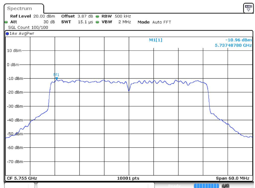
PSD ax40 5755MHz Ant1
