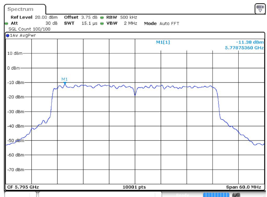
PSD ax40 5795MHz Ant1
