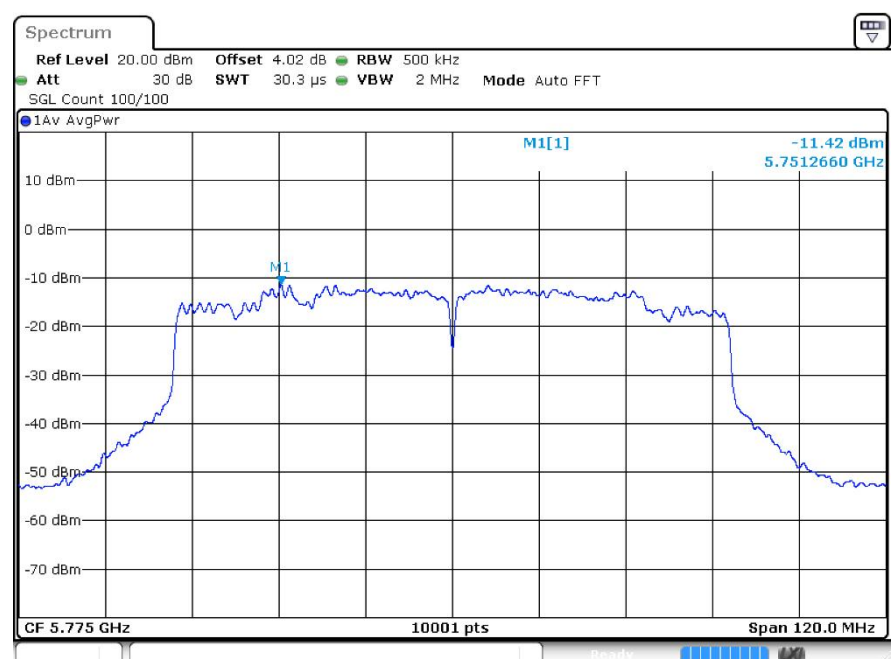
PSD ac80 5775MHz Ant2
