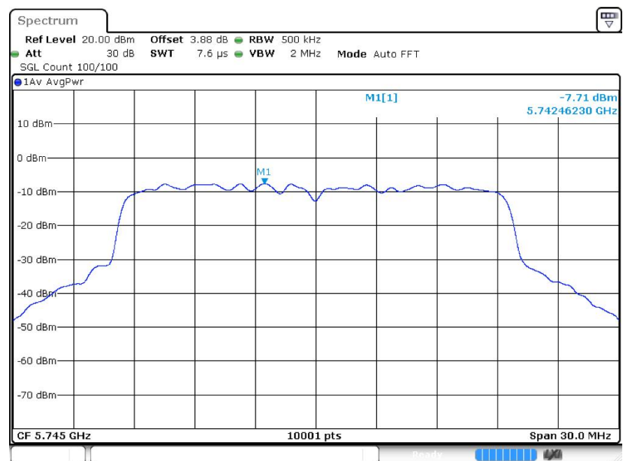
PSD ax20 5745MHz Ant1
