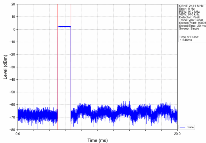
GFSK_DH3_HOPP_Ant1_NTNV
