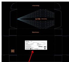
彩盒底贴标
